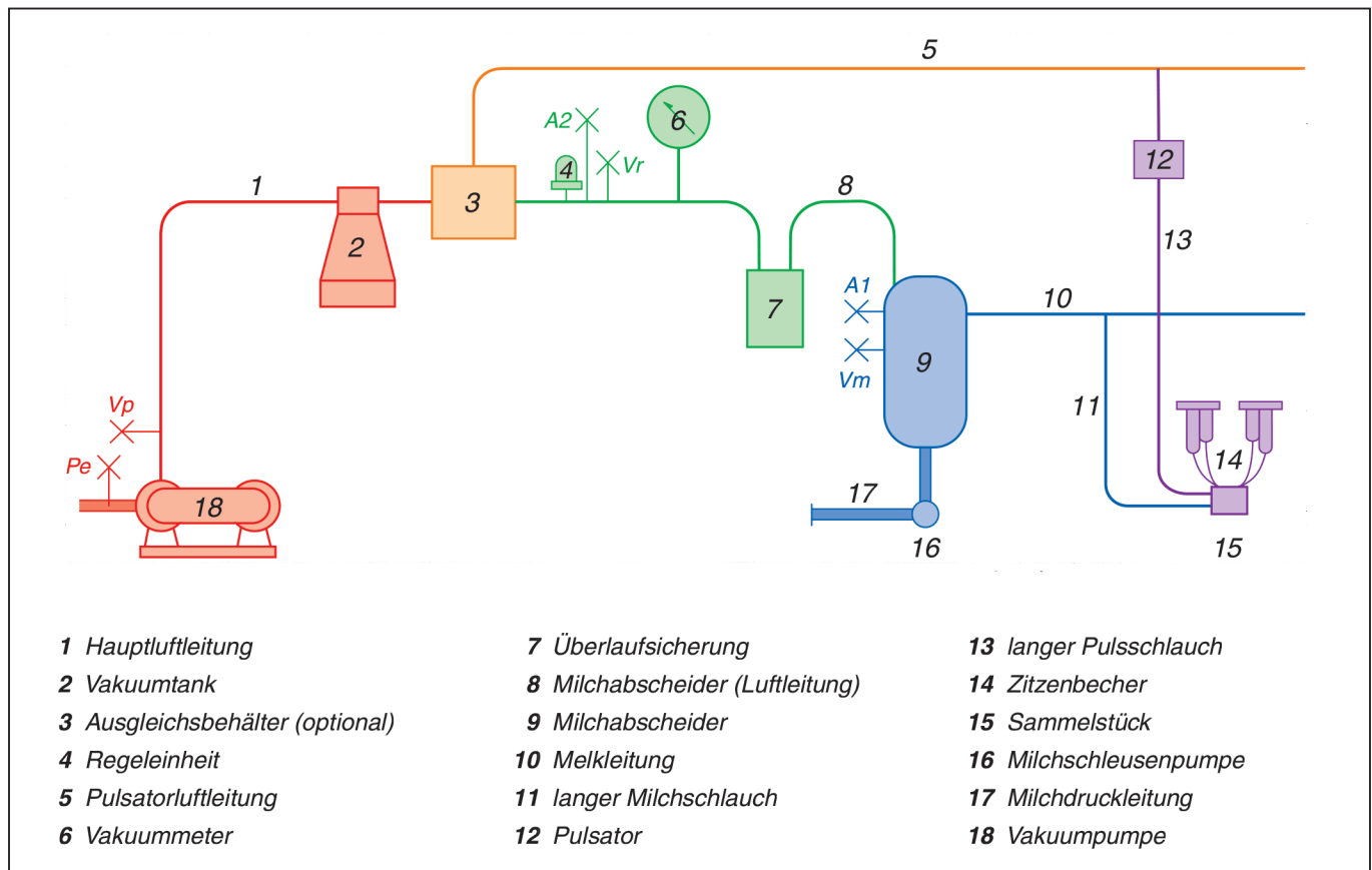
Abb. 16: Schema Melkanlage.
