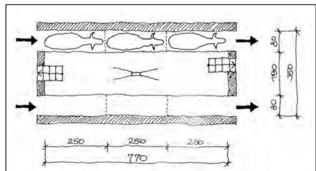
Abb. 27: Grundriss Durchtreibmelkstand.
