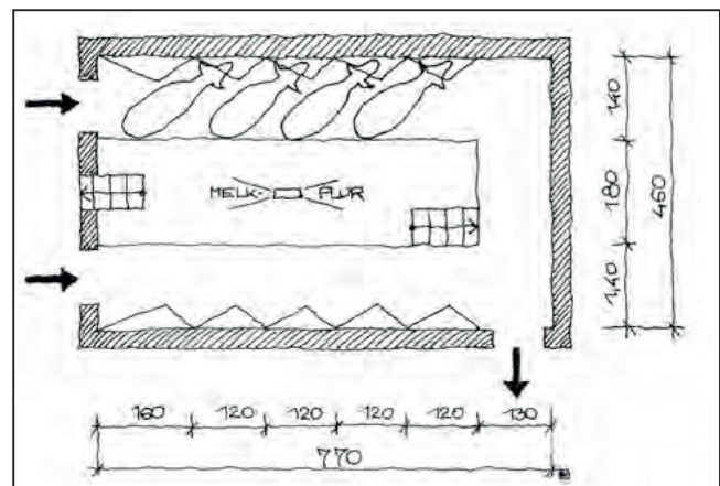
Abb. 26: Grundriss Fischgrätenmelkstand.
