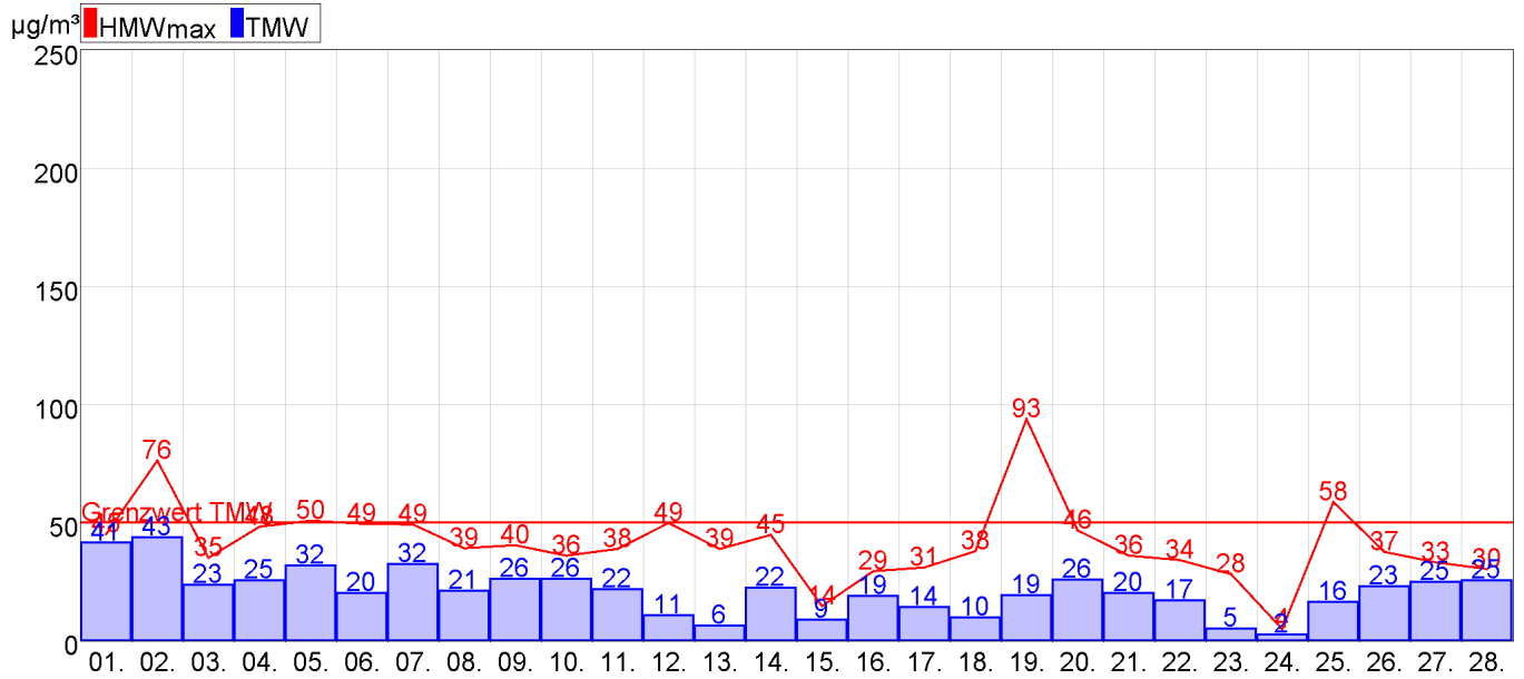
Abbildung 2: Eisenstadt PM10
