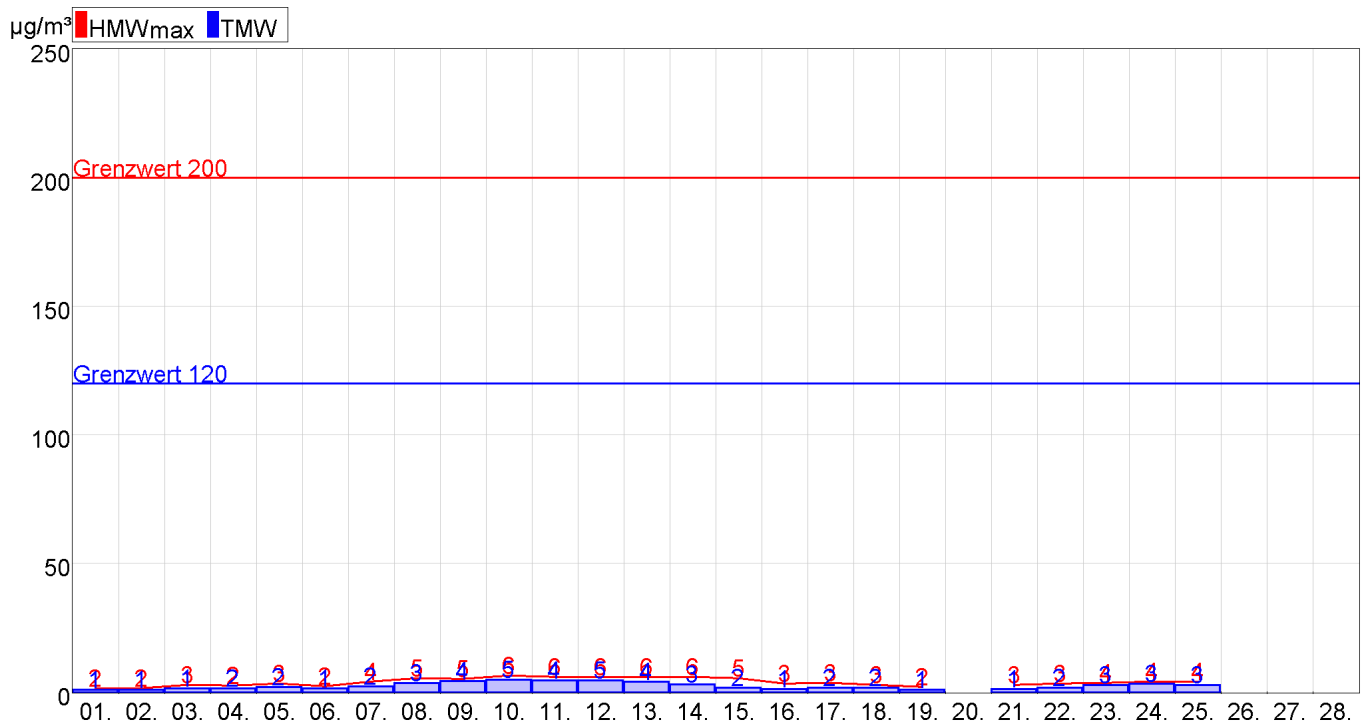
Abbildung 29: Rohr SO2
