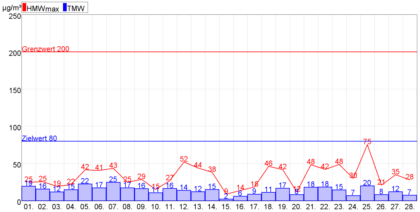
Abbildung 3: Eisenstadt NO2
