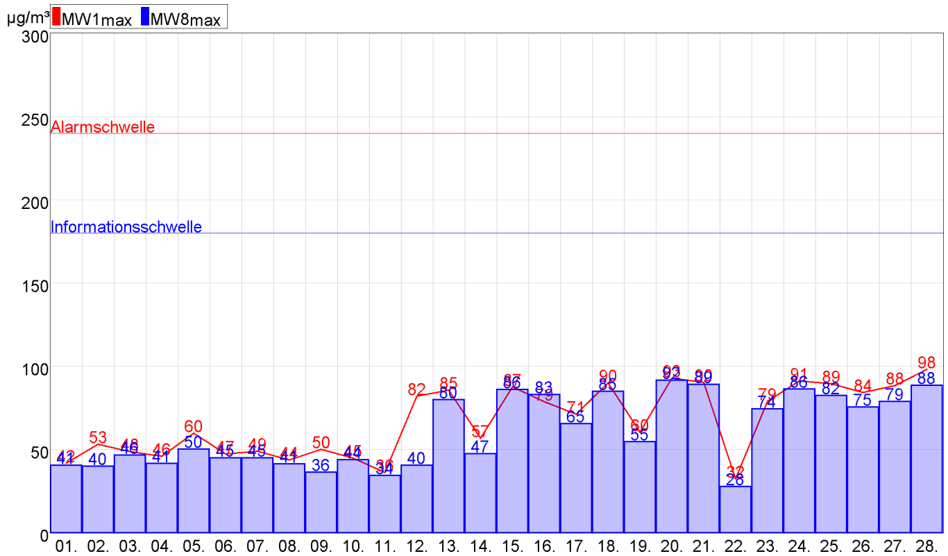
Abbildung 20: Kittsee O3
