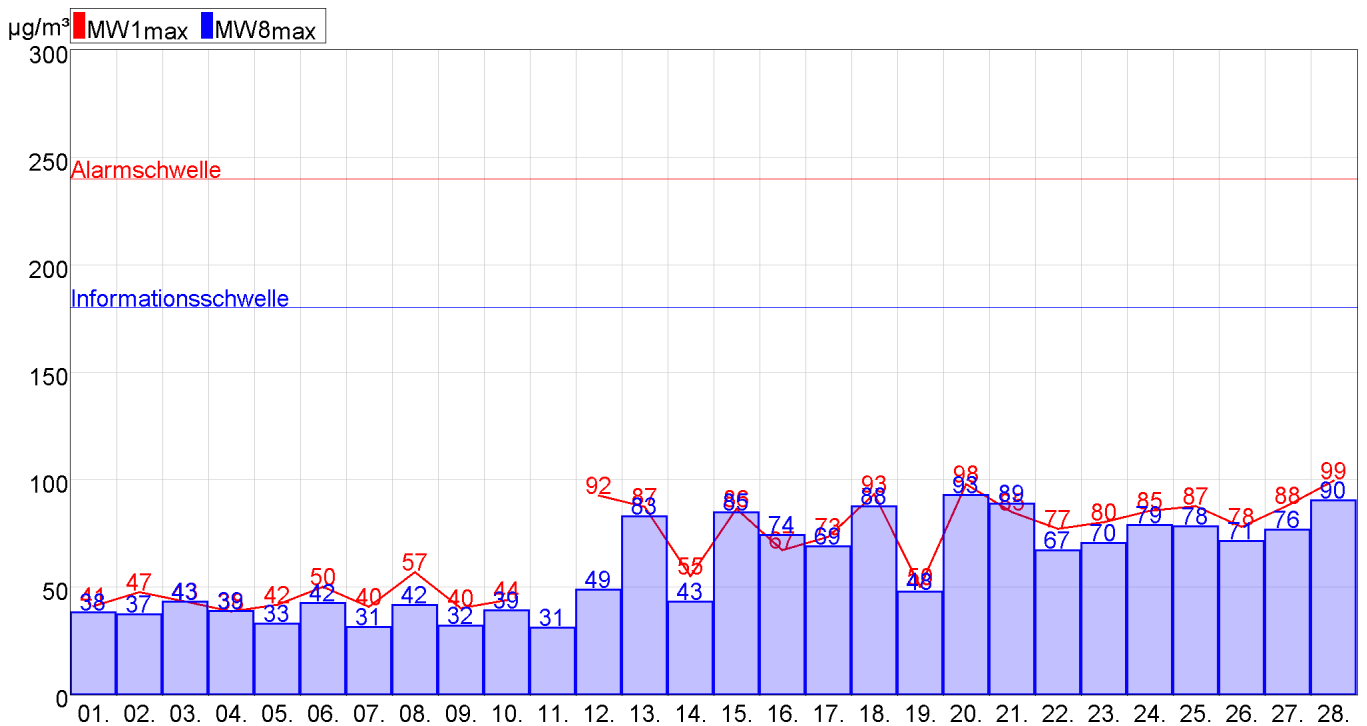
Abbildung 4: Eisenstadt O3
