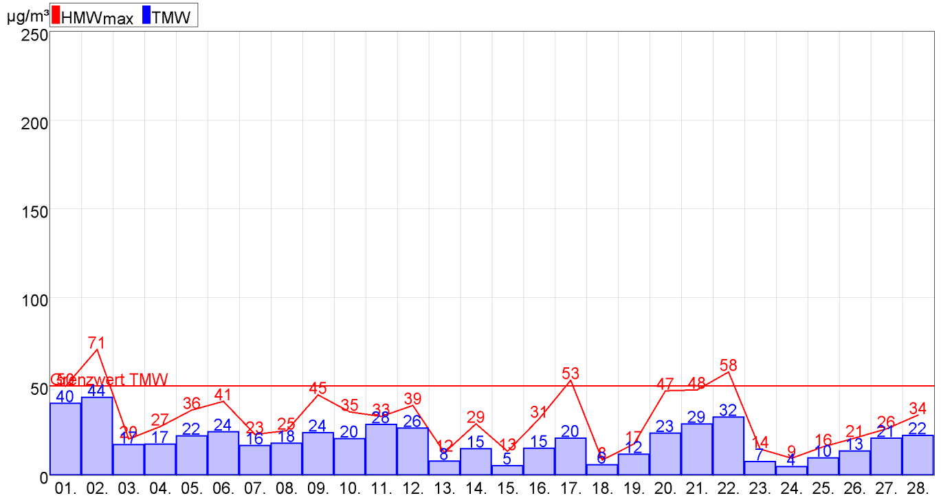
Abbildung 18: Kittsee PM10
