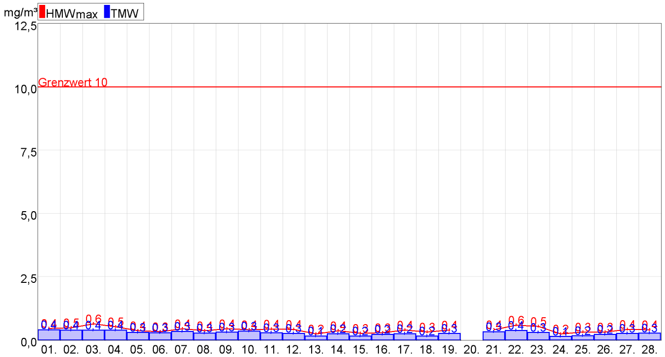
Abbildung 30: Rohr CO
