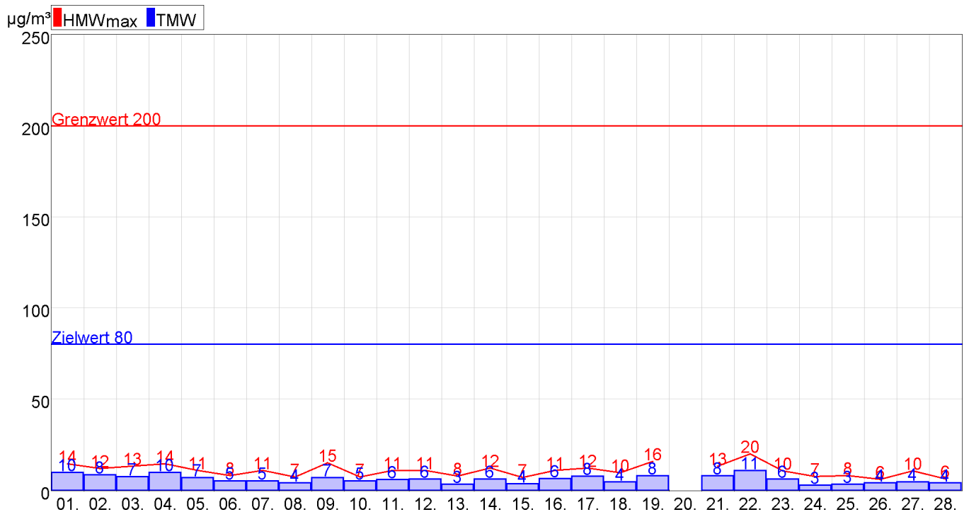
Abbildung 27: Rohr NO2
