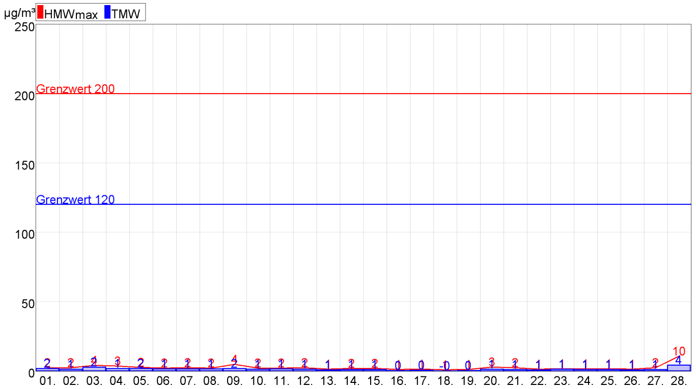
Abbildung 5: Eisenstadt SO2
