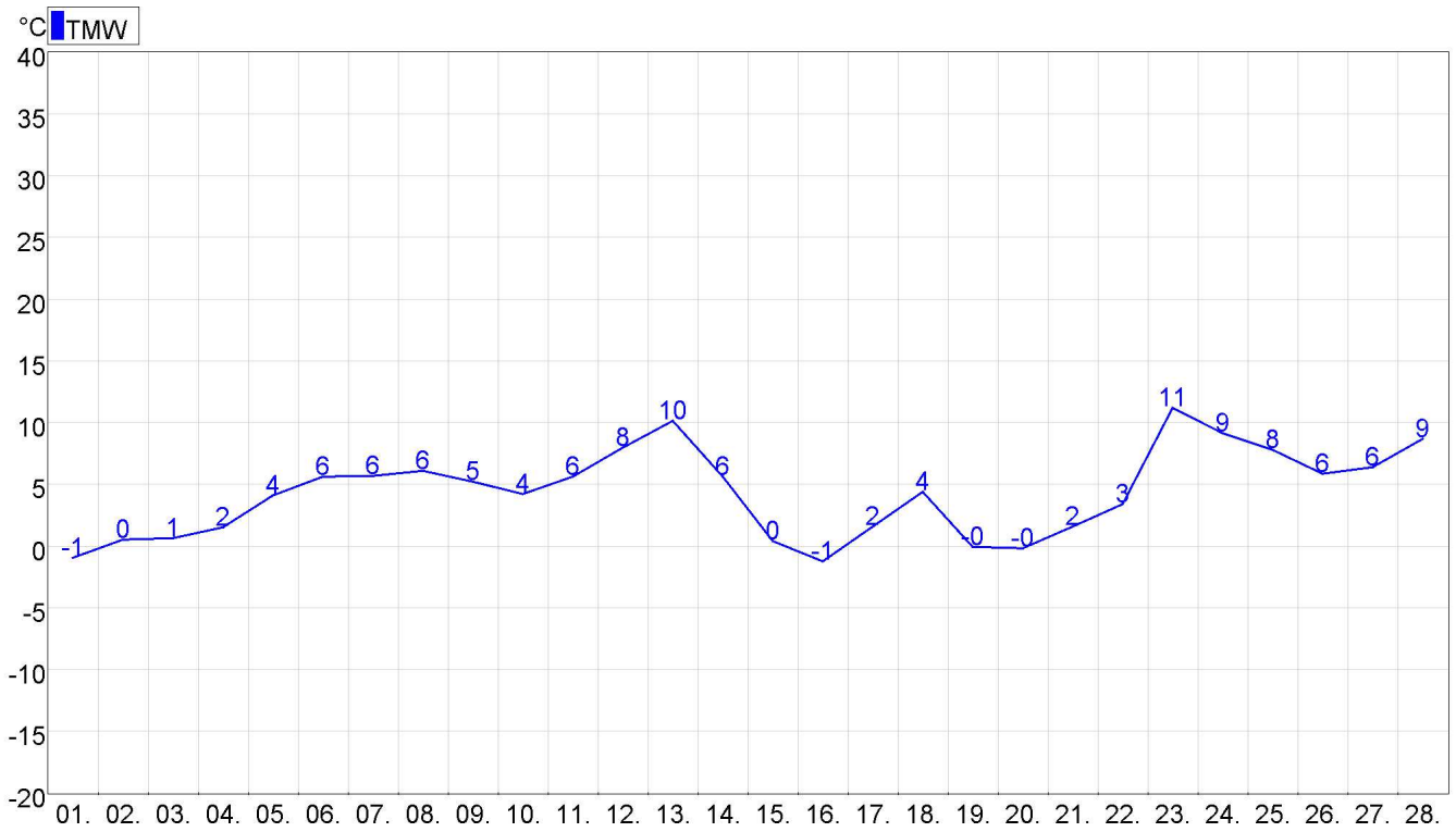
Abbildung 7: Eisenstadt Lufttemperatur
