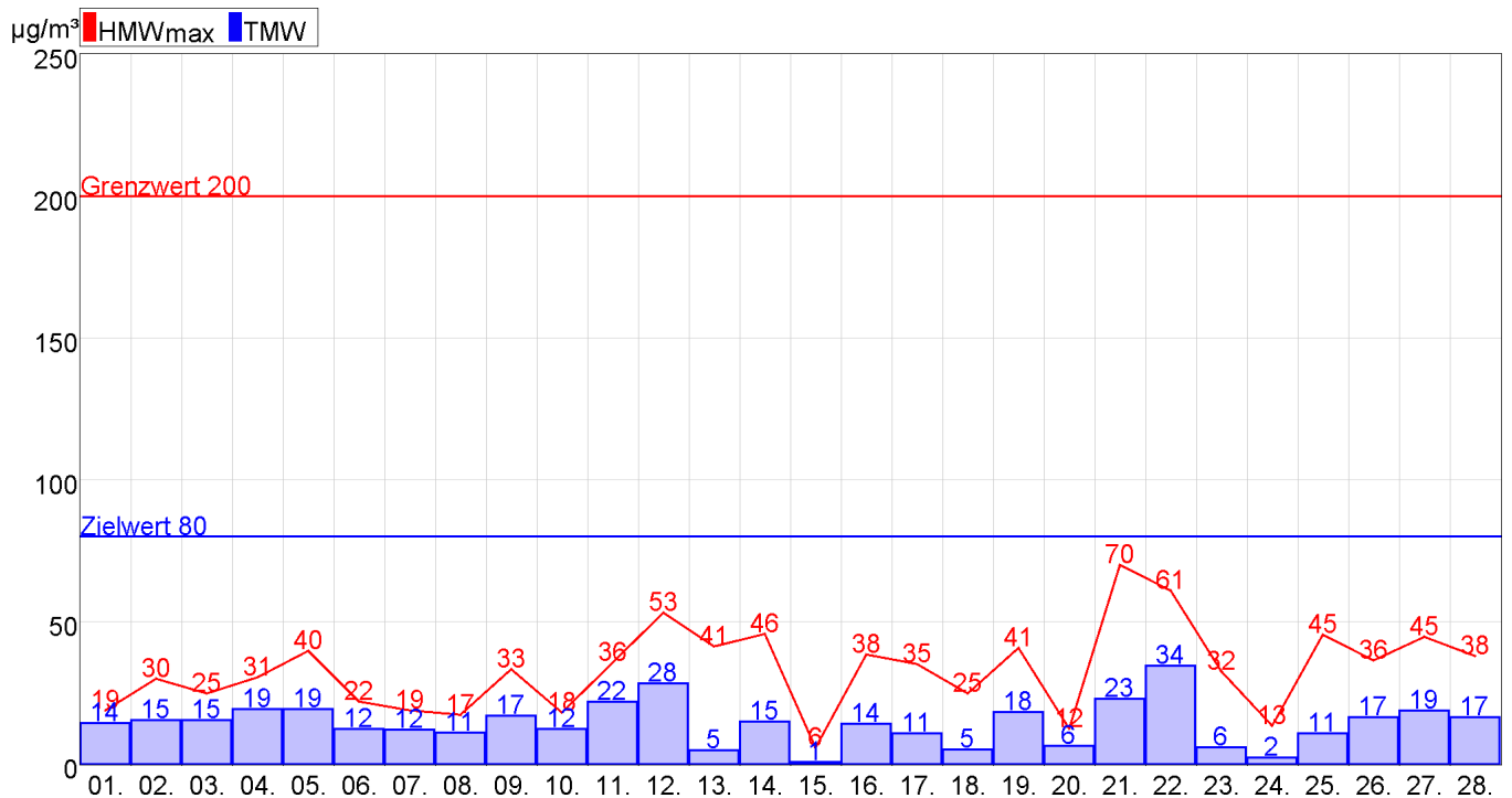
Abbildung 19: Kittsee NO2
