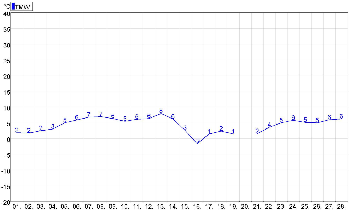
Abbildung 31: Rohr Lufttemperatur
