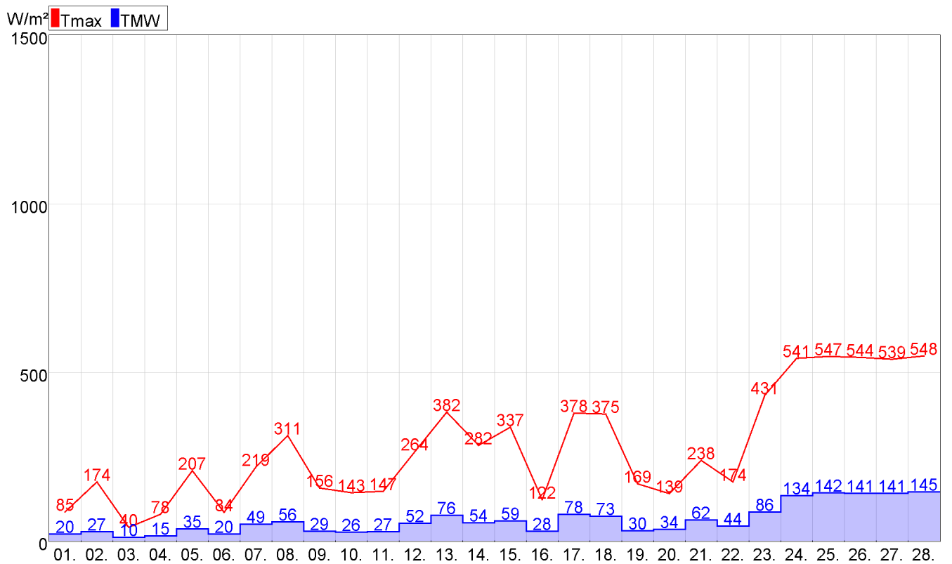
Abbildung 25: Kittsee Globalstrahlung
