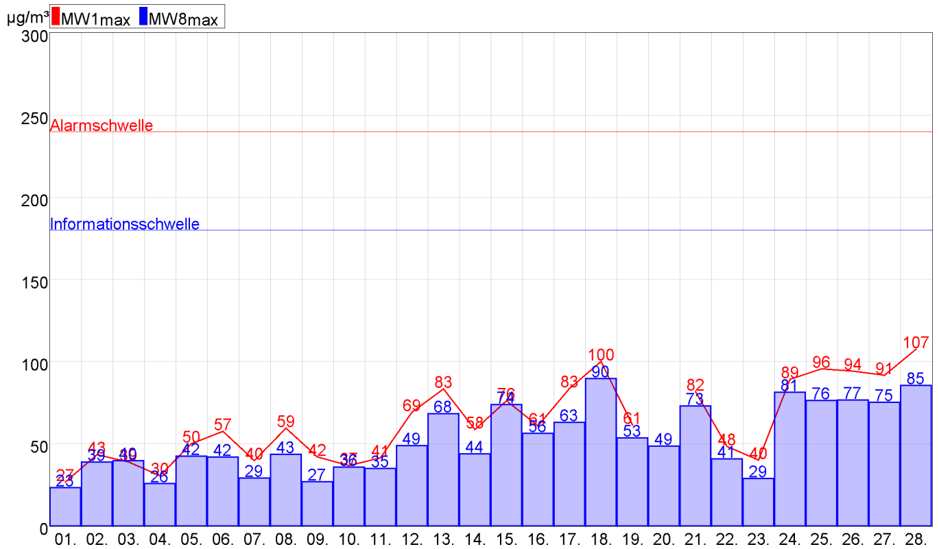
Abbildung 28: Rohr O3
