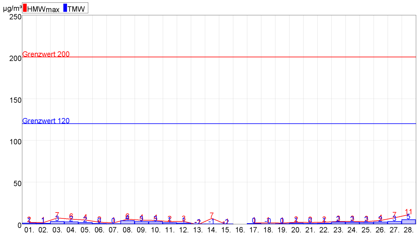
Abbildung 21: Kittsee SO2
