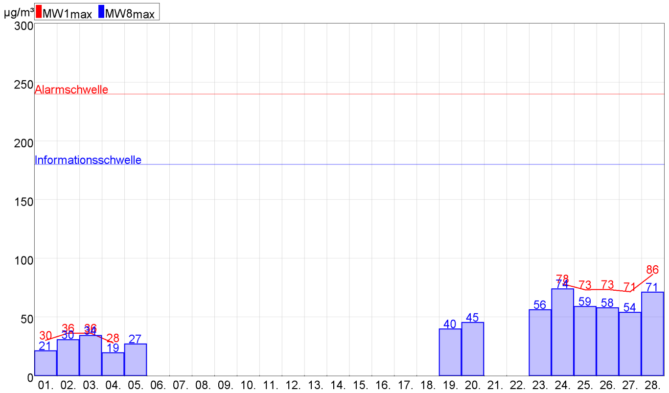
Abbildung 13: Oberwart O3
