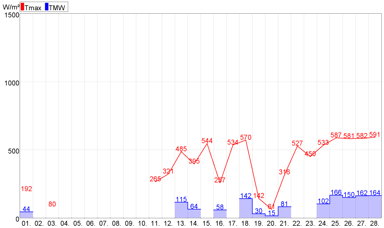
Abbildung 17: Oberwart Globalstrahlung
