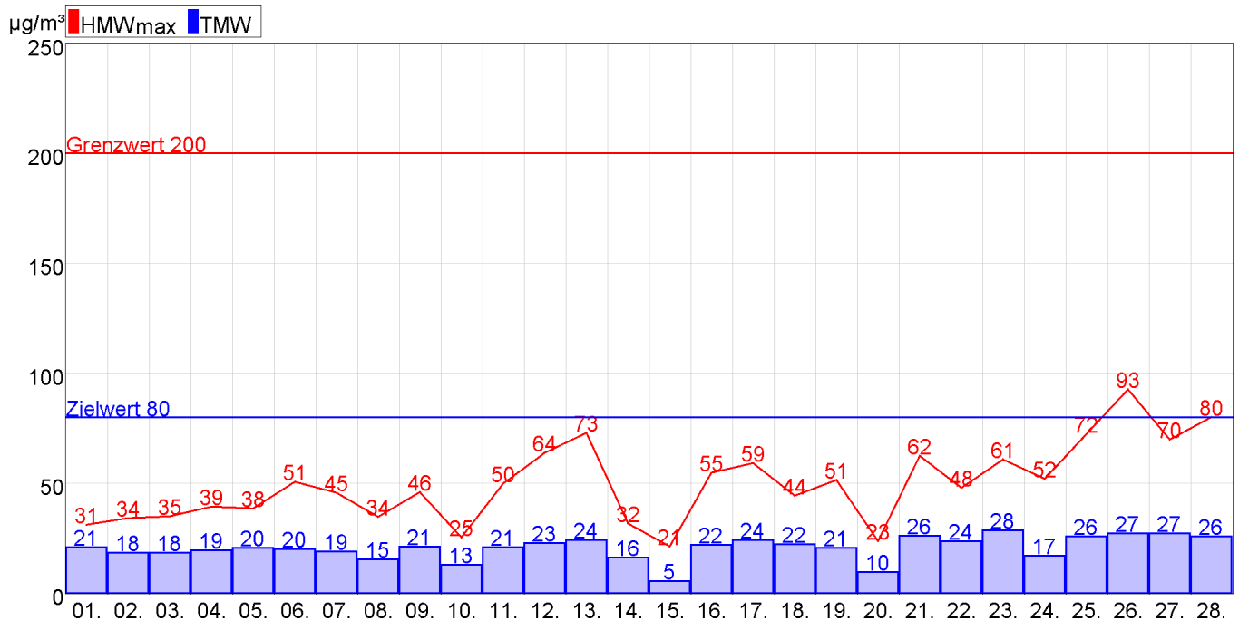
Abbildung 12: Oberwart NO2
