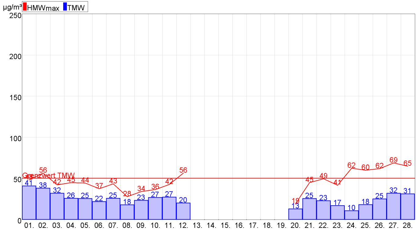
Abbildung 11: Oberwart PM10
