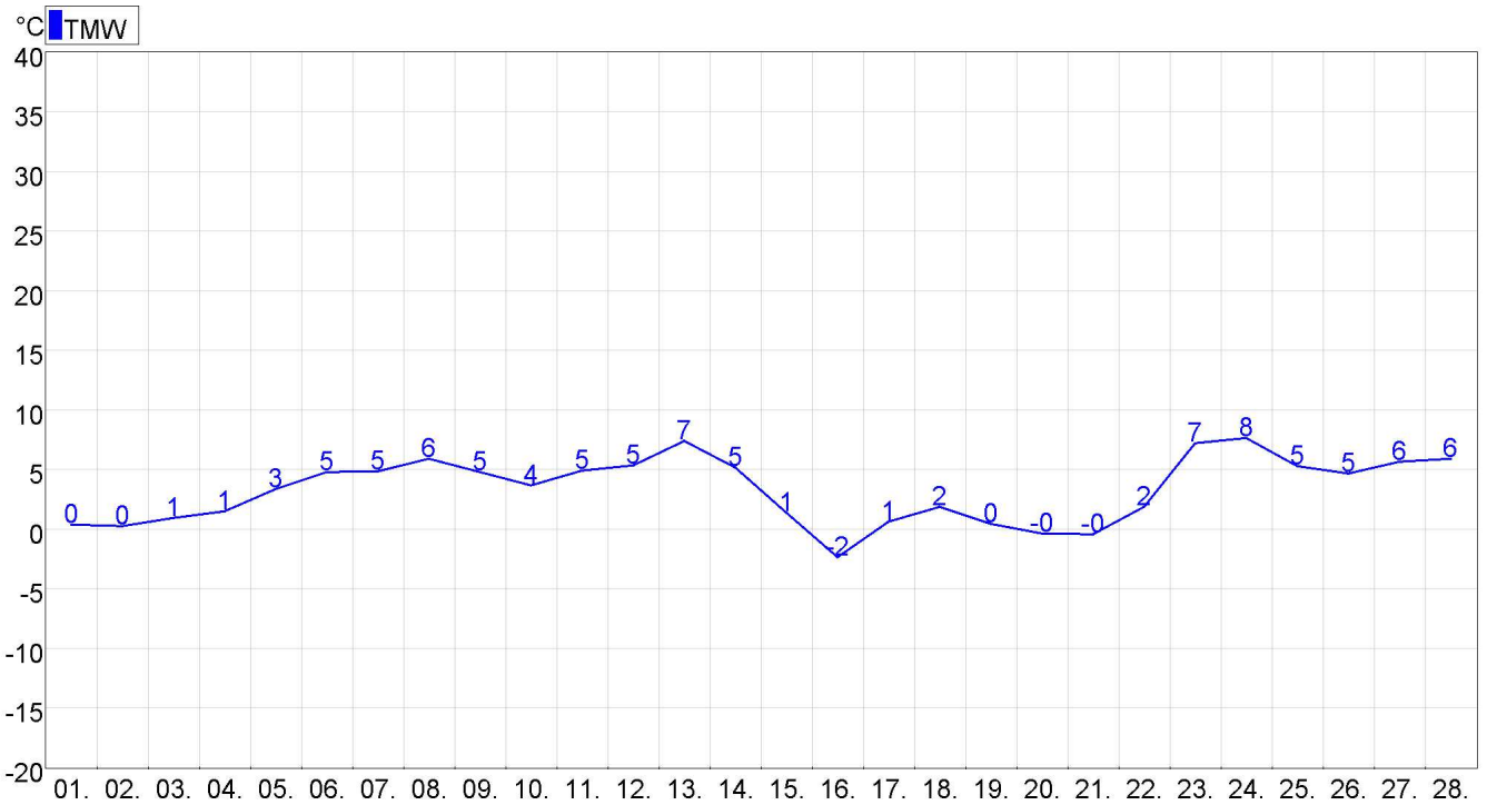
Abbildung 14: Oberwart Lufttemperatur
