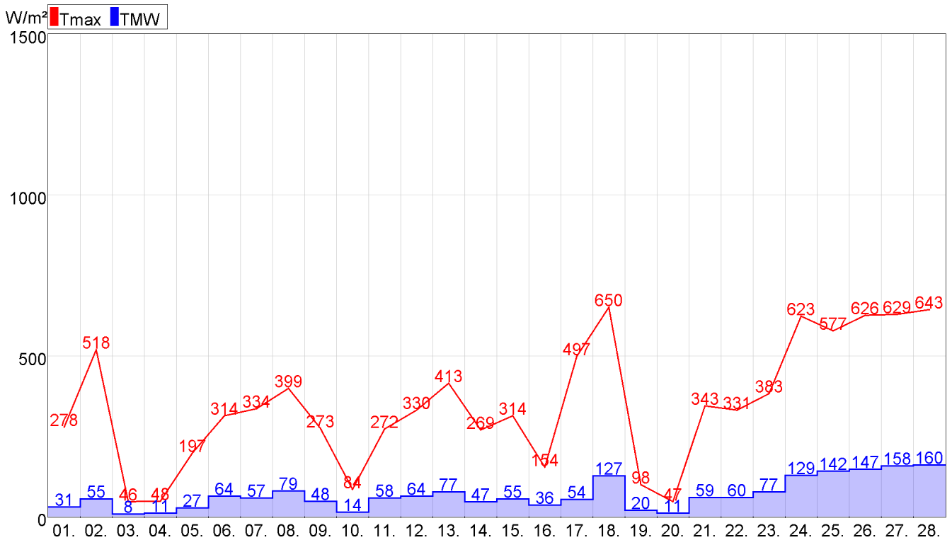
Abbildung 10: Eisenstadt Globalstrahlung
