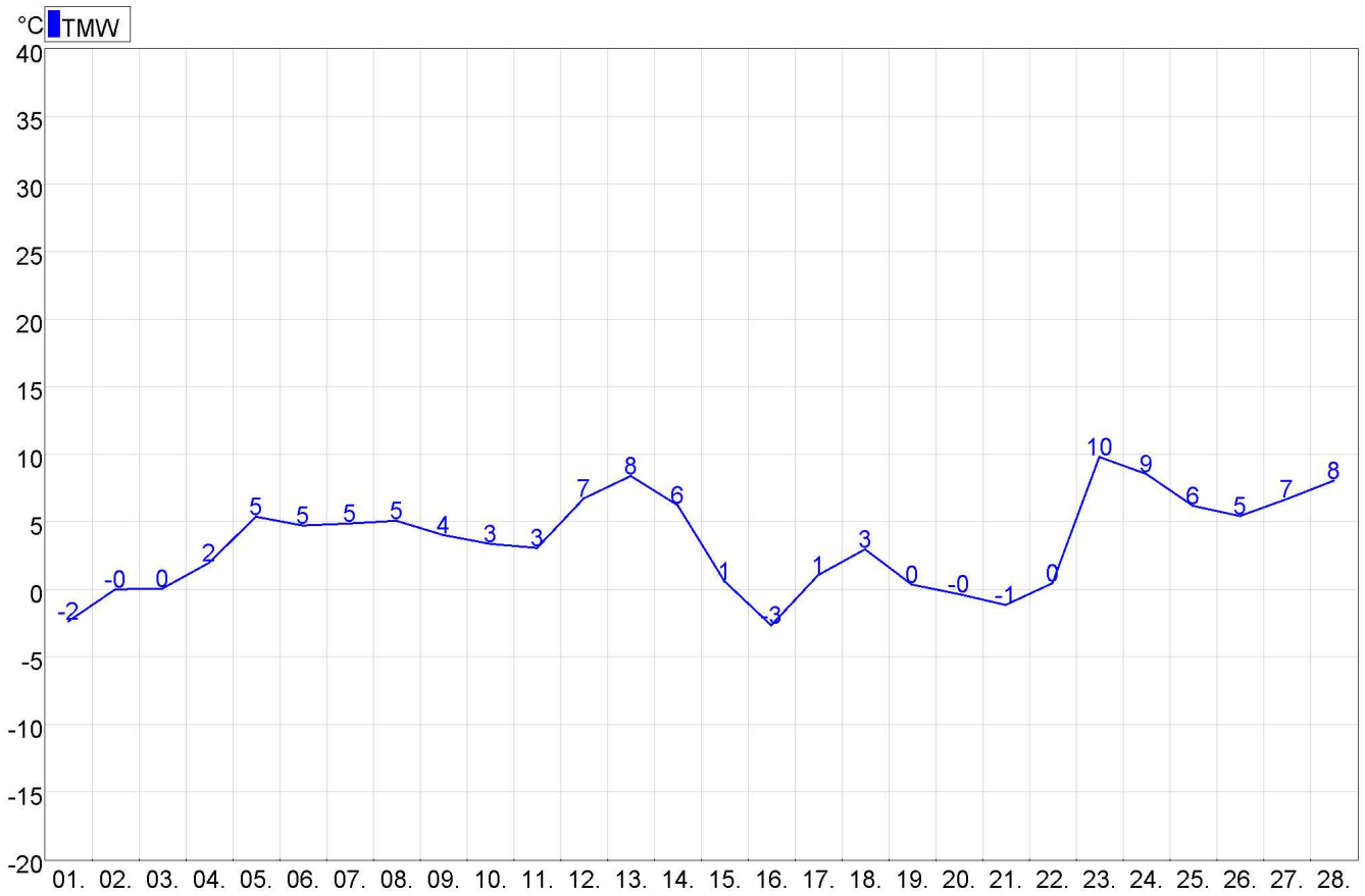
Abbildung 22: Kittsee Lufttemperatur
