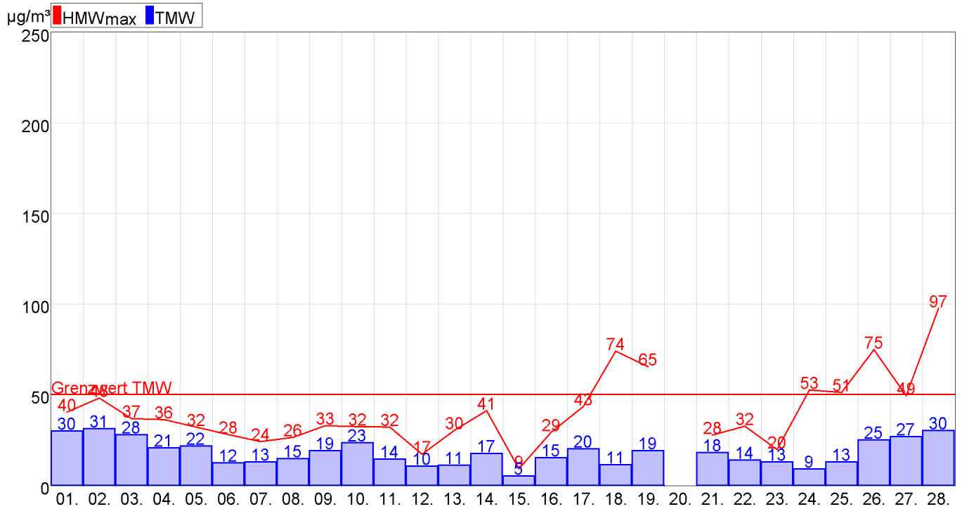
Abbildung 26: Rohr PM10
