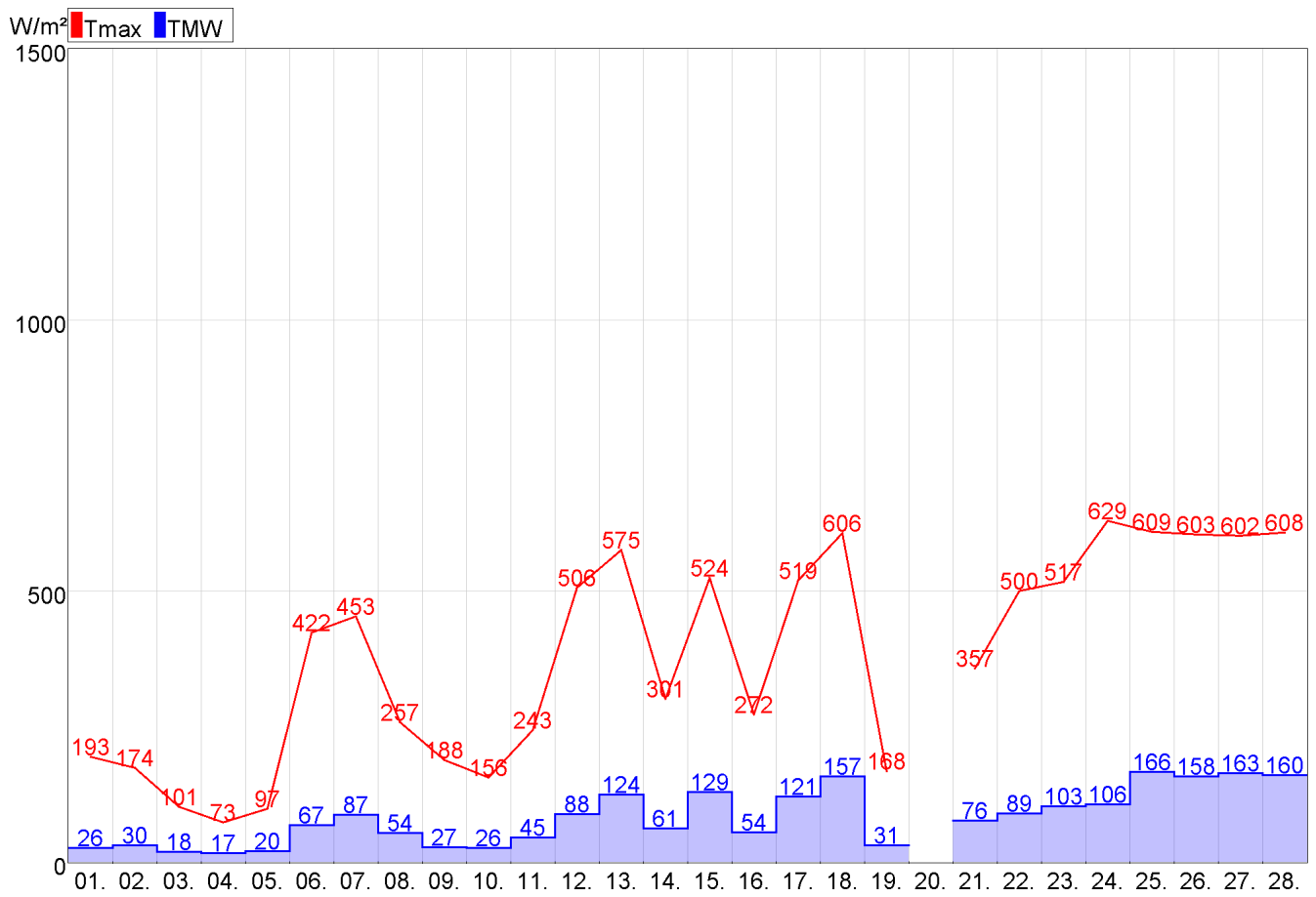
Abbildung 34: Rohr Globalstrahlung
