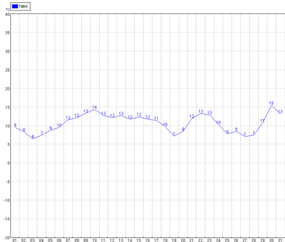
Abbildung 31: Rohr Lufttemperatur
