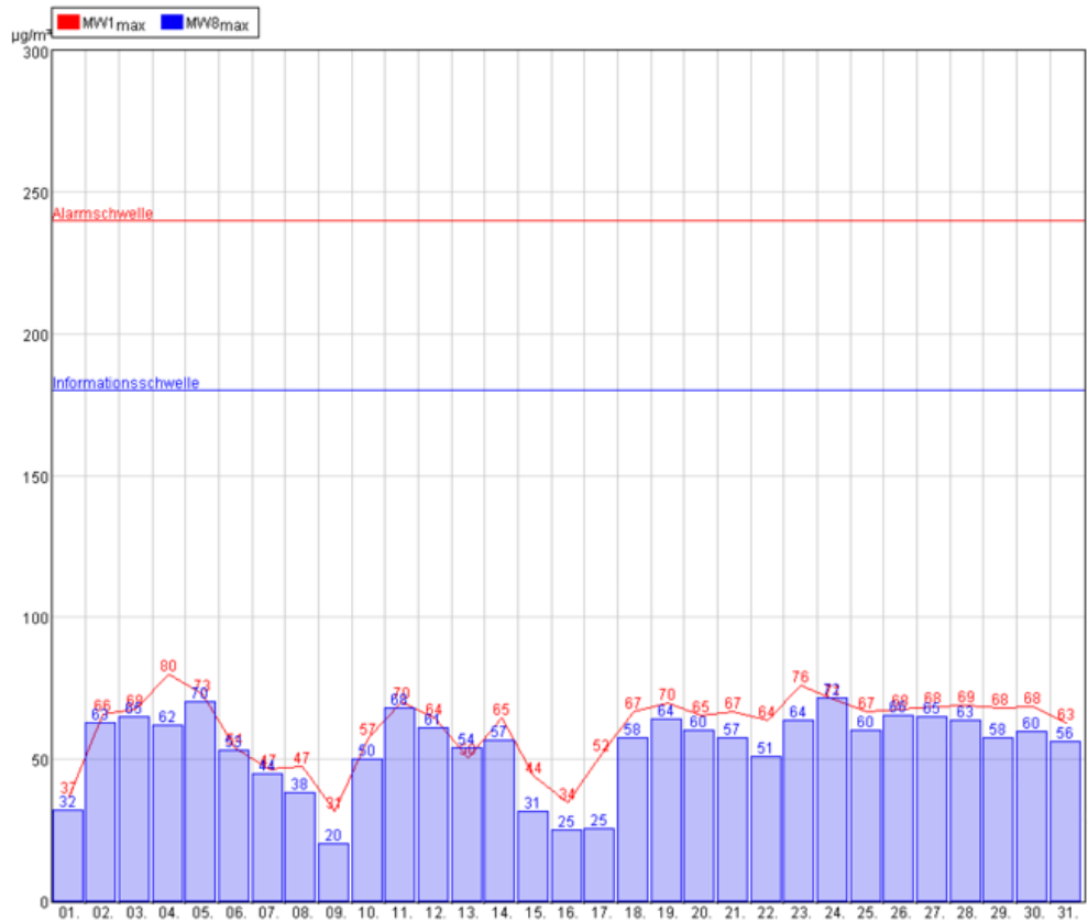
Abbildung 4: Eisenstadt O 3
