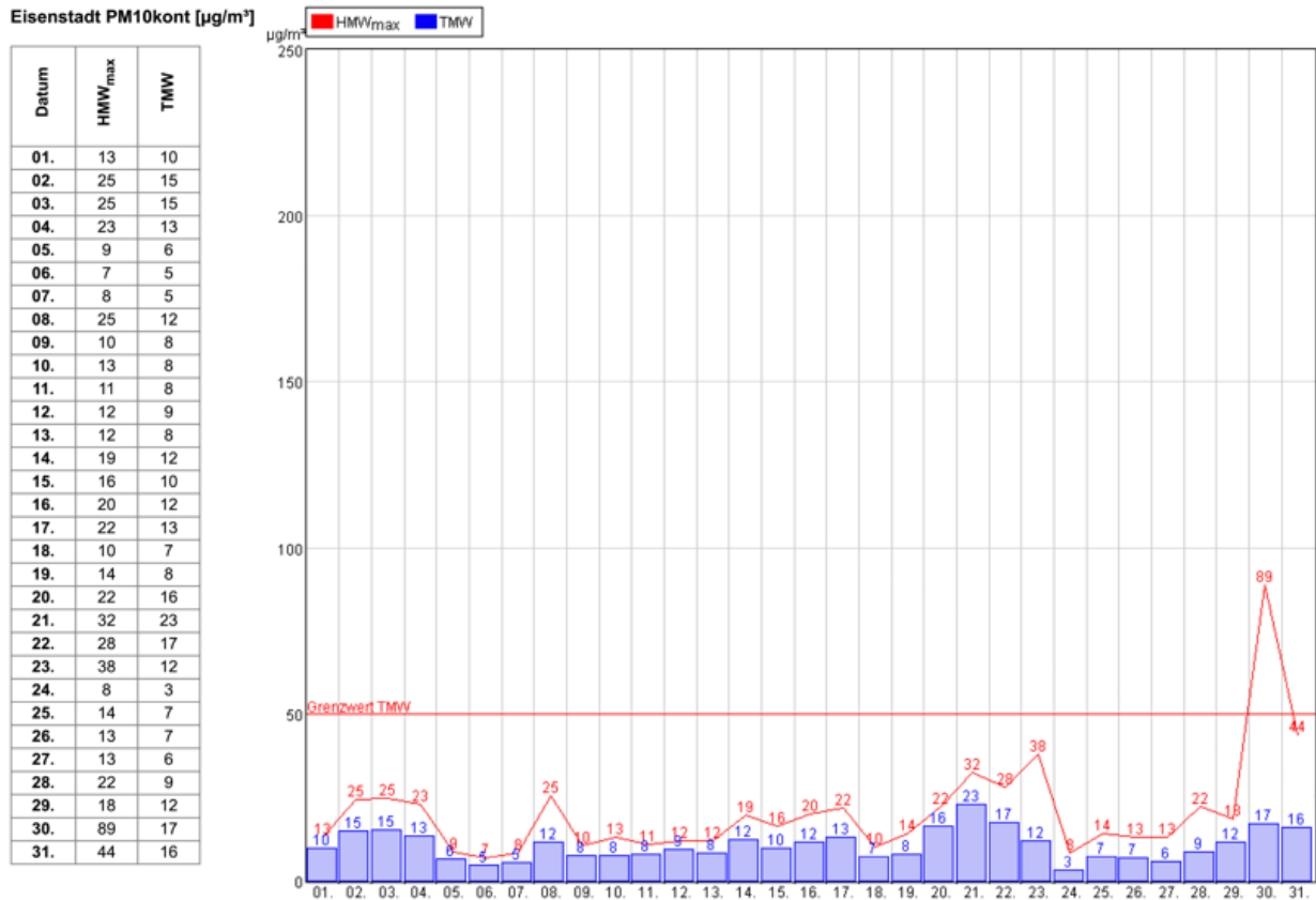
Abbildung 2: Eisenstadt PM 10
