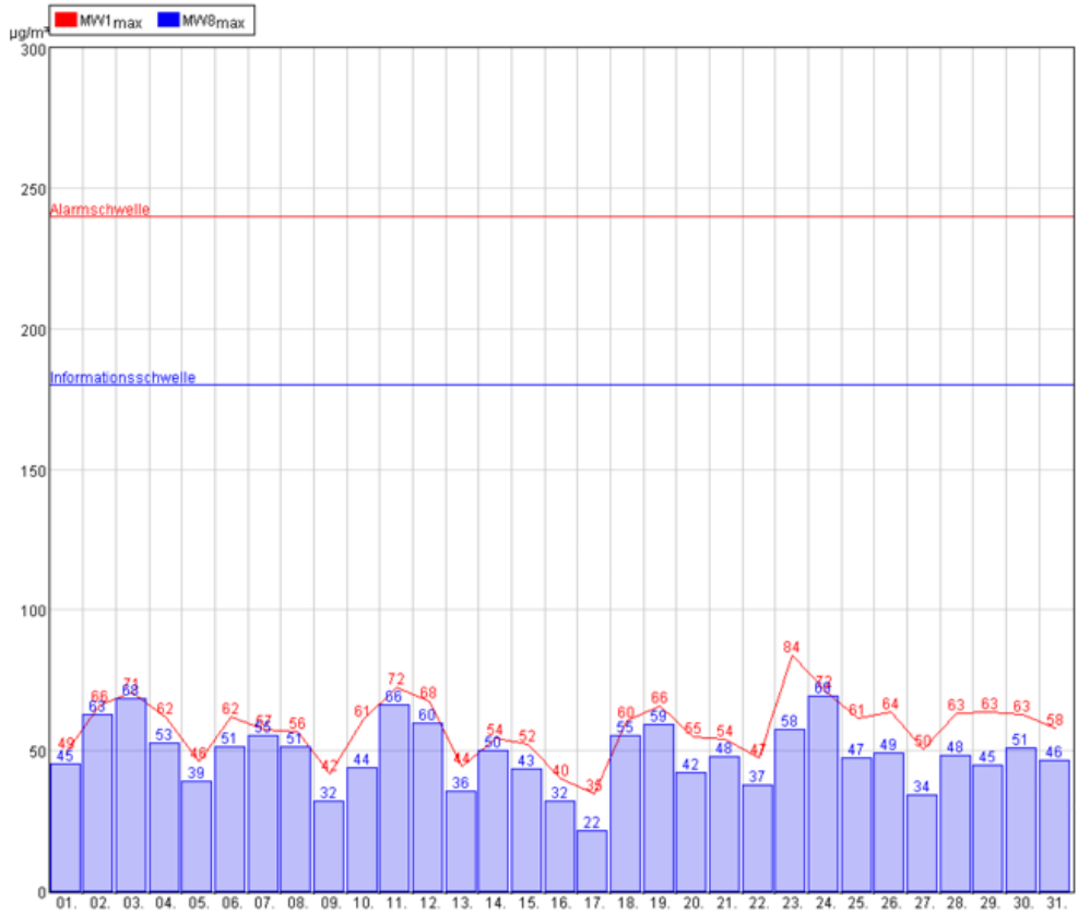
Abbildung 13: Oberwart O 3
