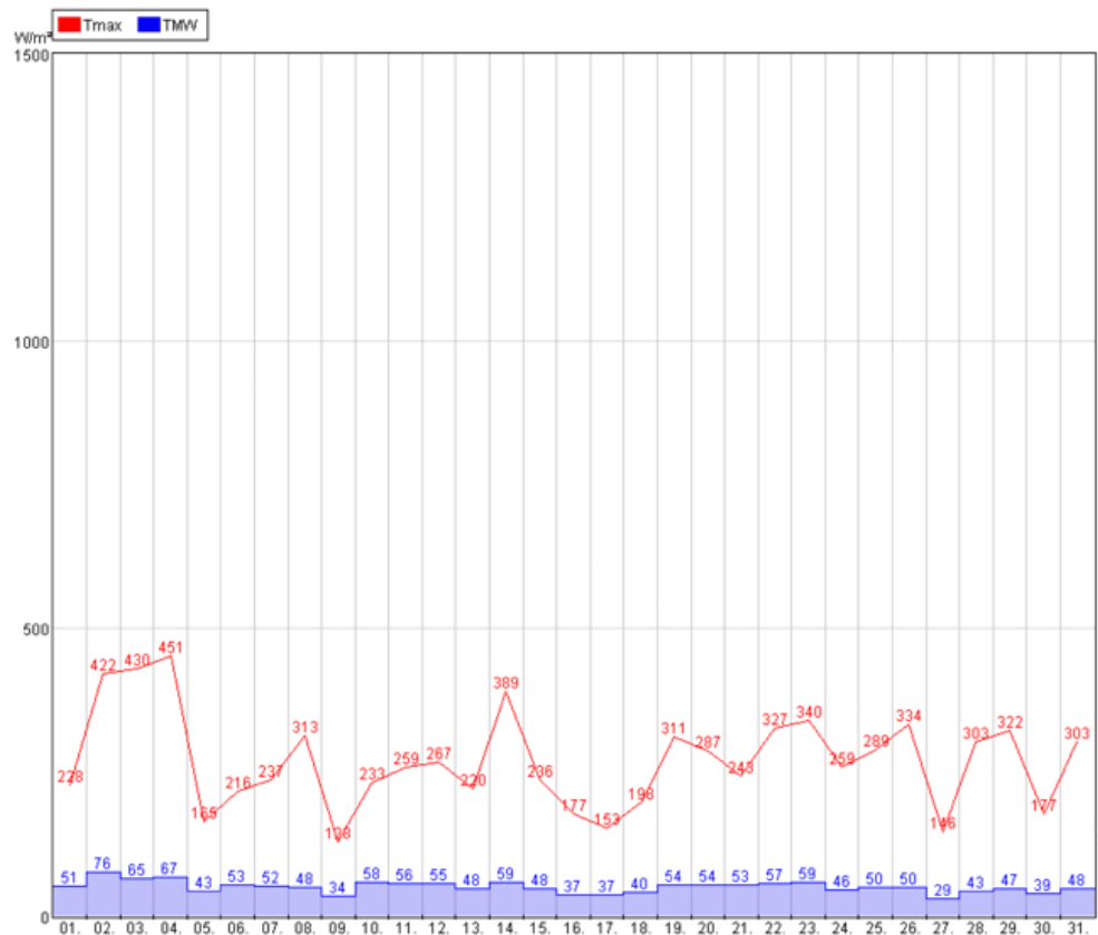
Abbildung 10: Eisenstadt Globalstrahlung
