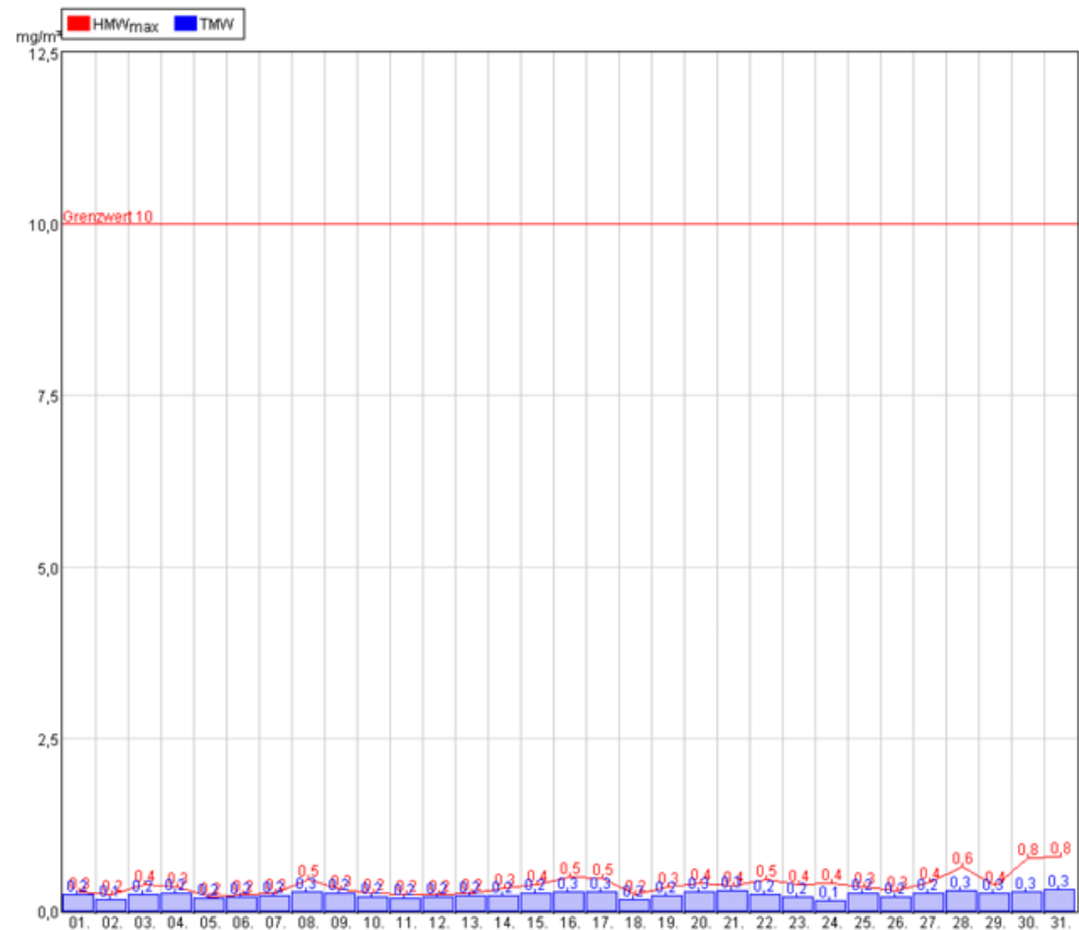
Abbildung 6: Eisenstadt CO
