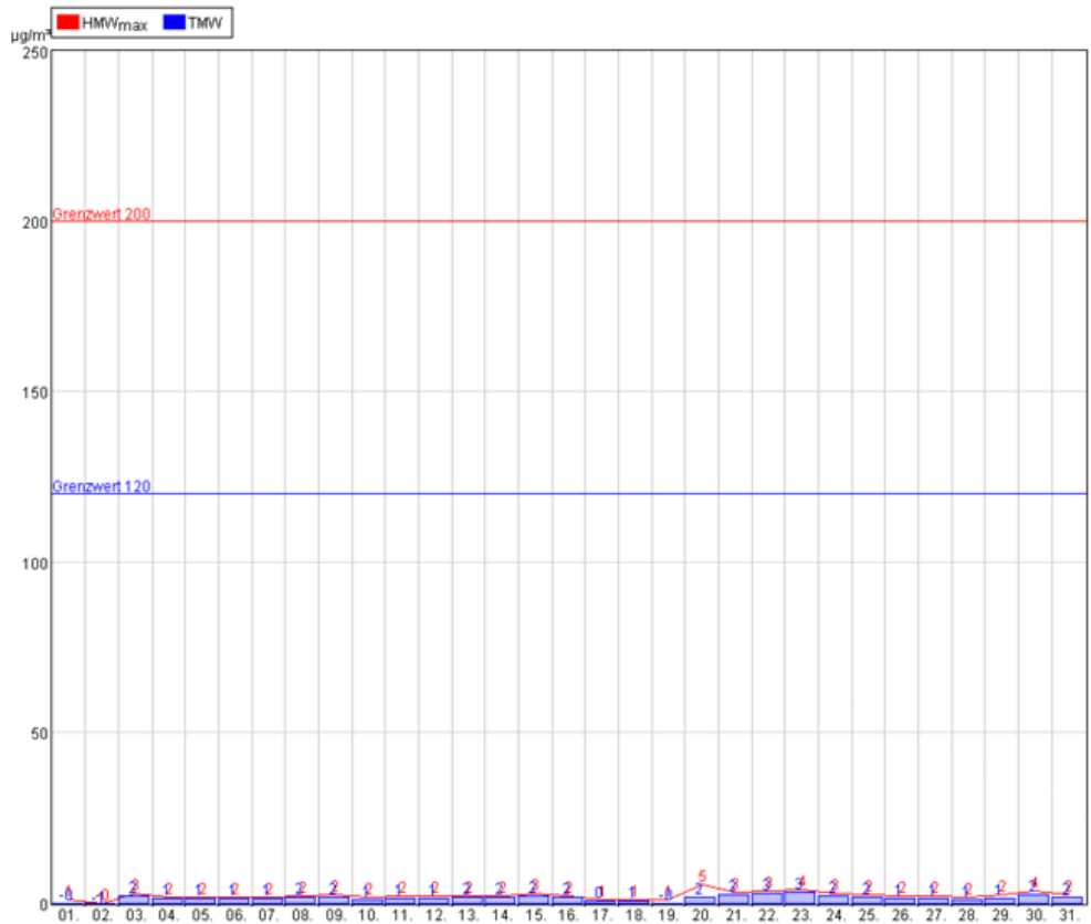
Abbildung 29: Rohr SO 2
