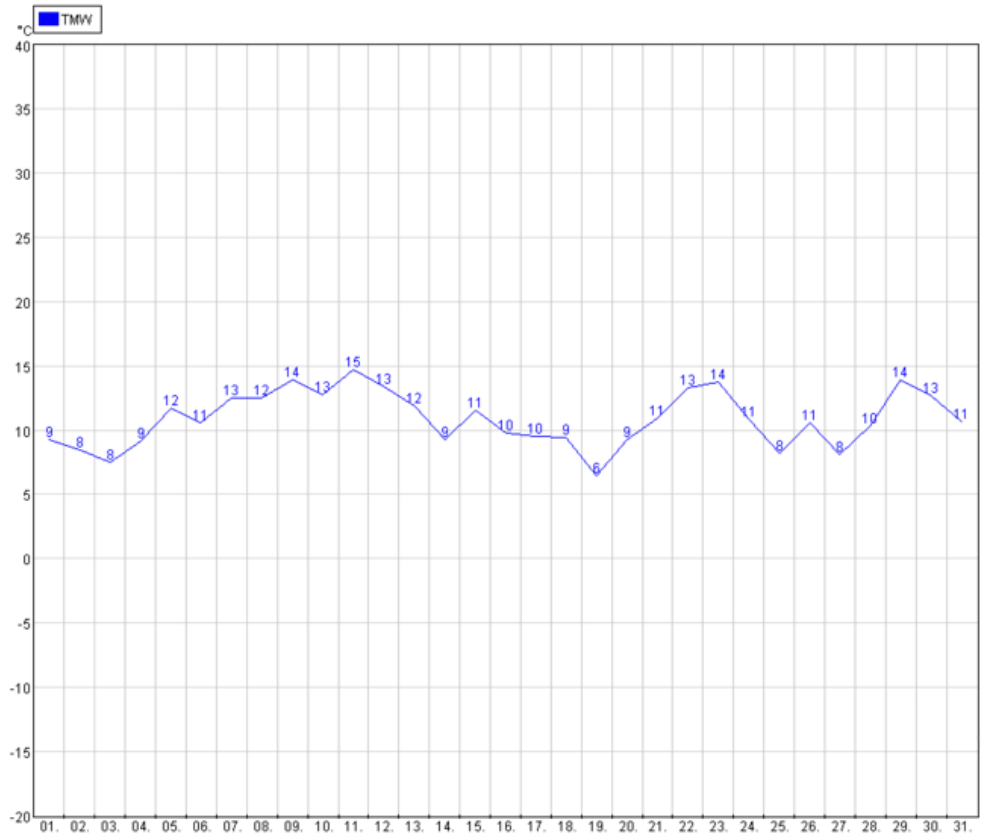
Abbildung 22: Kittsee Lufttemperatur
