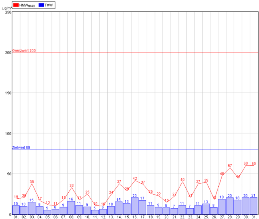
Abbildung 3: Eisenstadt NO 2
