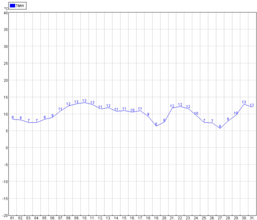
Abbildung 14: Oberwart Lufttemperatur
