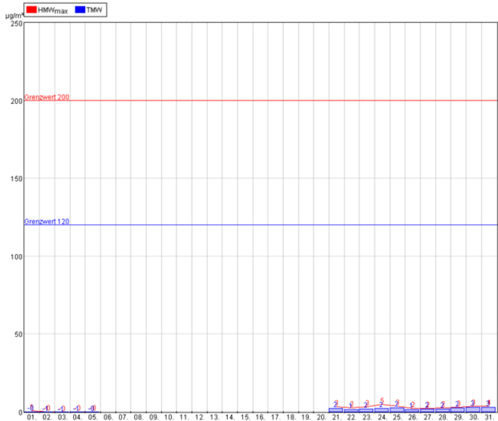
Abbildung 5: Eisenstadt SO 2
