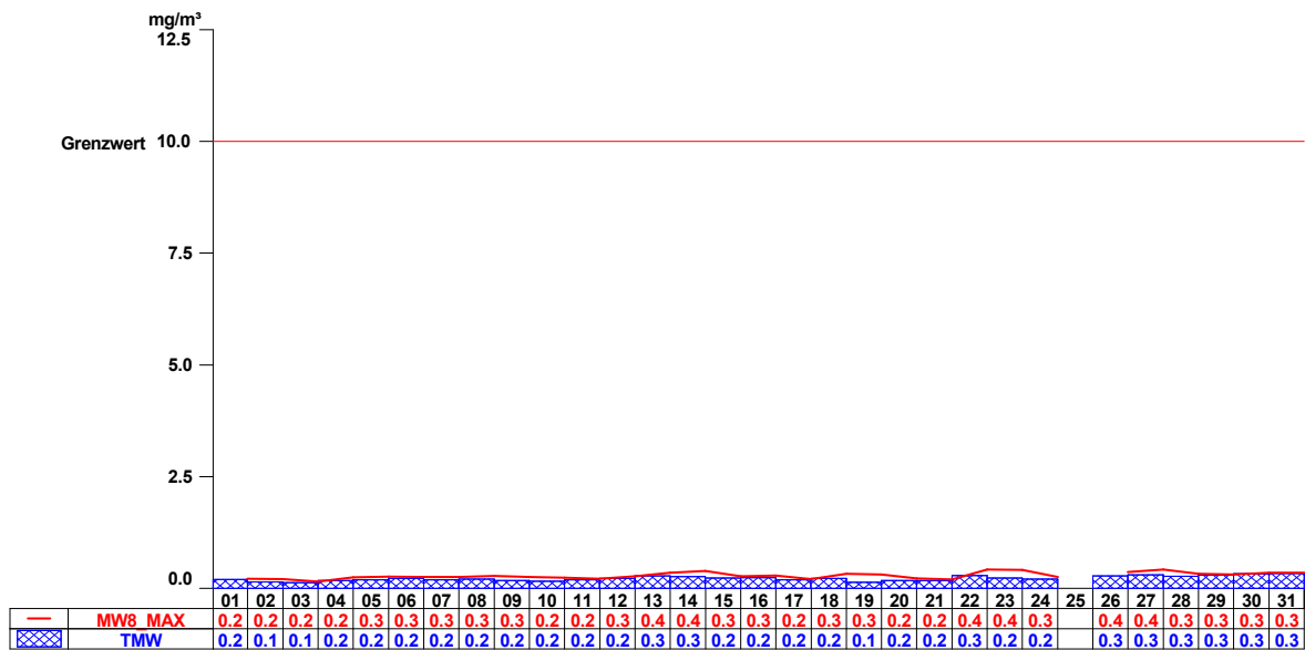
Abbildung 5: Eisenstadt CO
