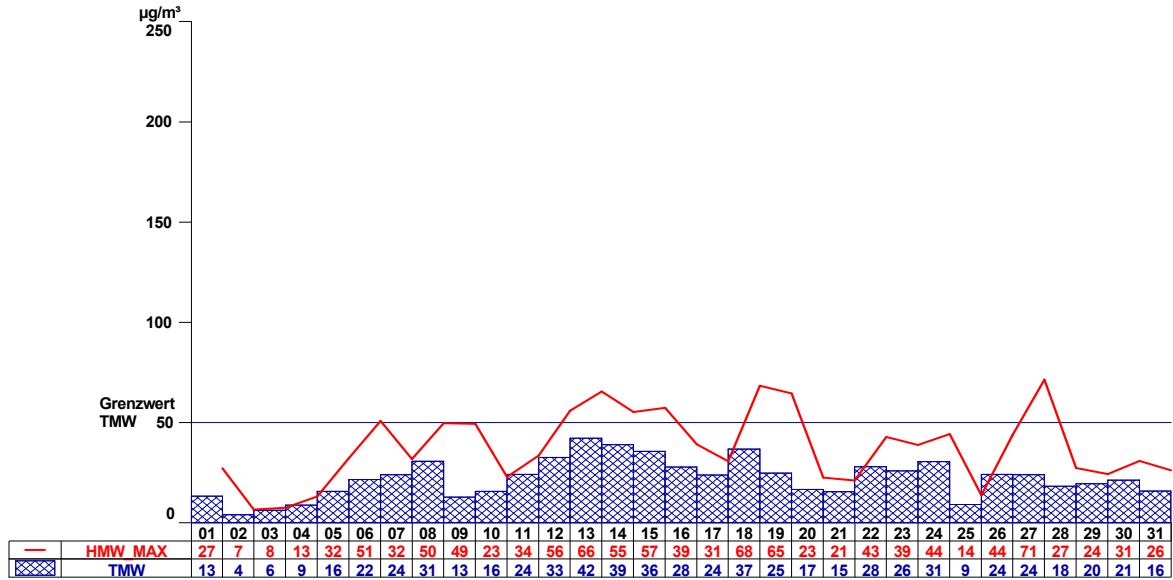
Abbildung 20: Kittsee PM 10
