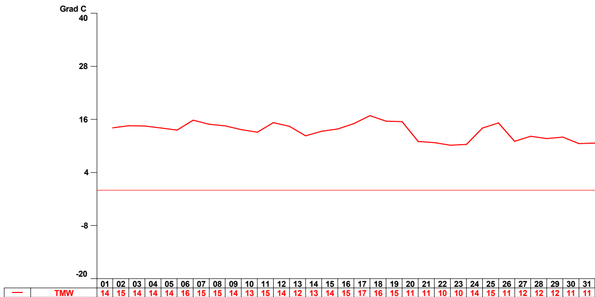
Abbildung 7: Eisenstadt Lufttemperatur
