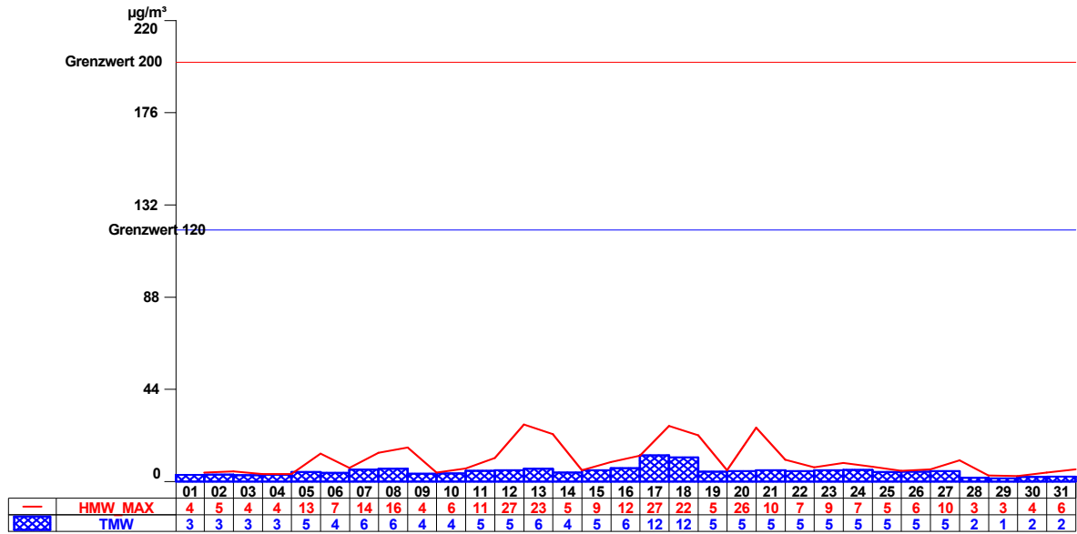
Abbildung 18: Kittsee SO 2
