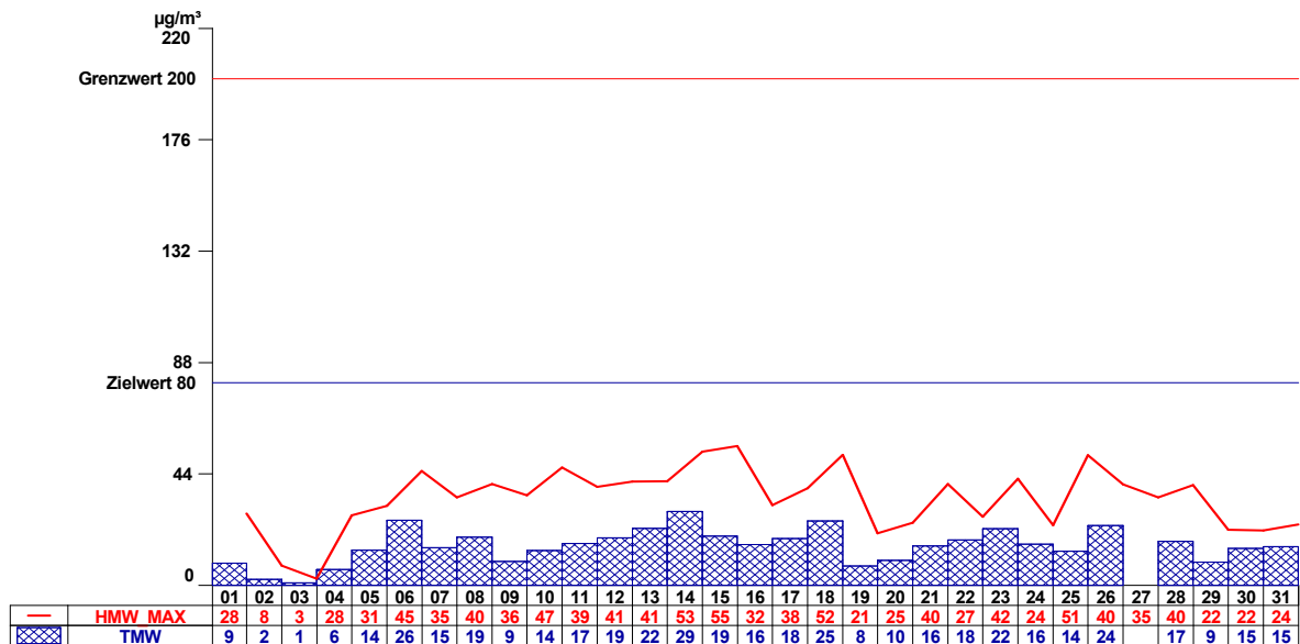
Abbildung 19: Kittsee NO 2
