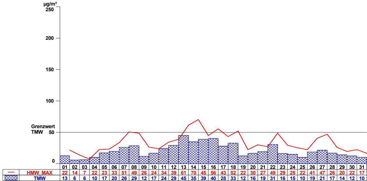
Abbildung 4: Eisenstadt PM 10
