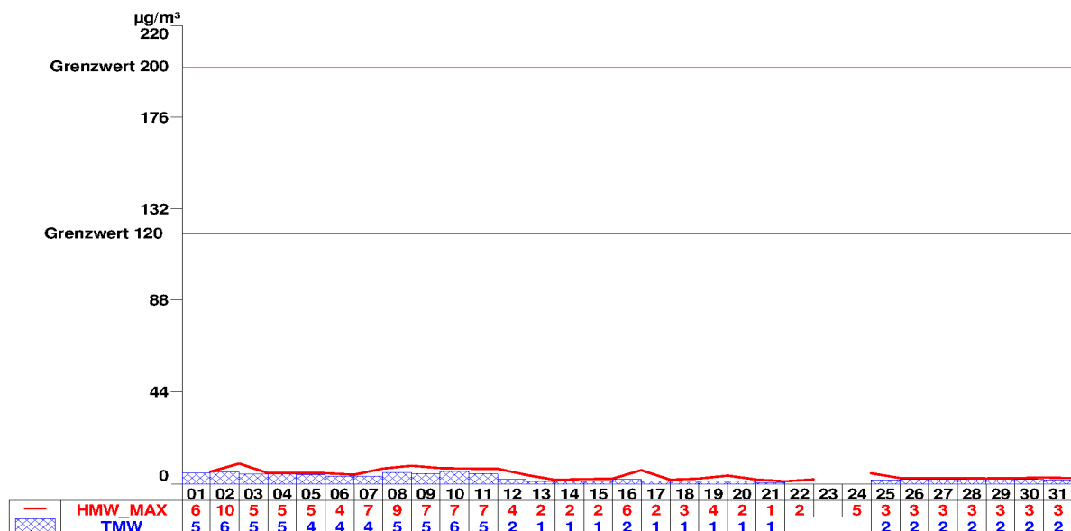
Abbildung 18: Kittsee SO 2
