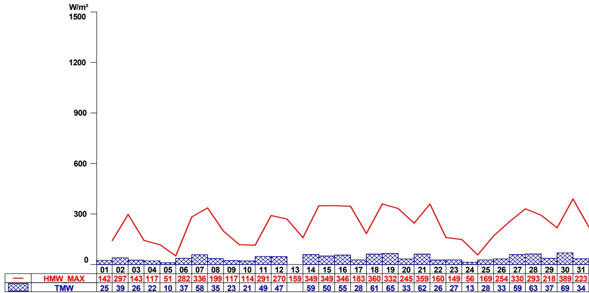
Abbildung 10: Eisenstadt Globalstrahlung
