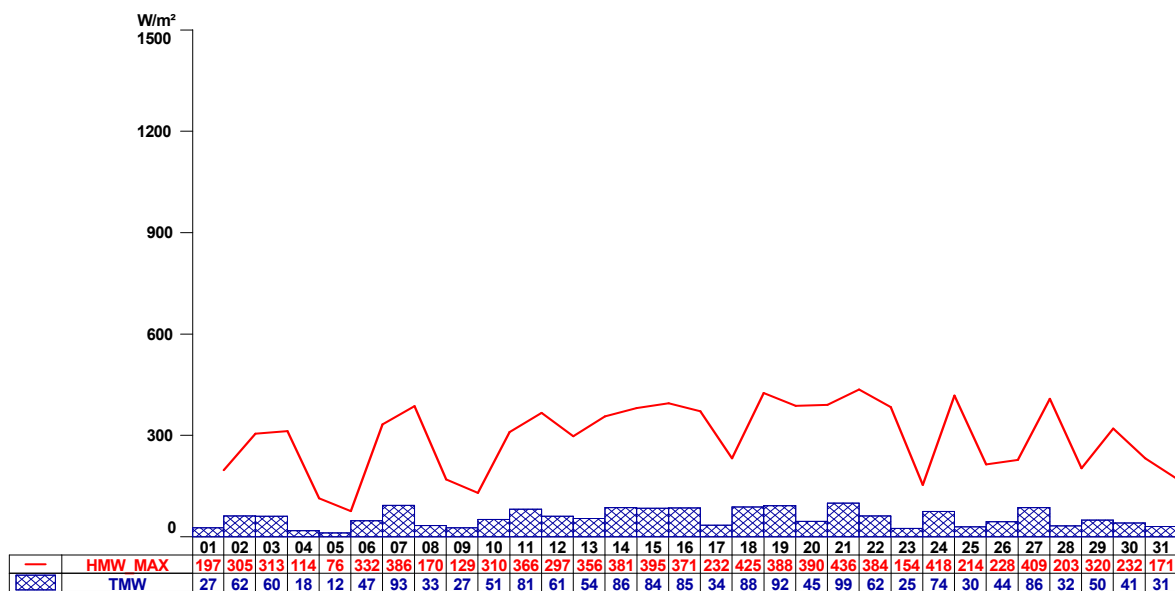
Abbildung 25: Kittsee Globalstrahlung
