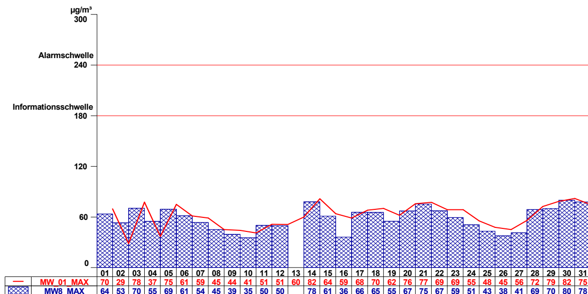
Abbildung 6: Eisenstadt O 3
