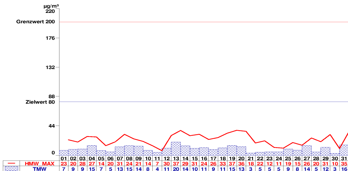
Abbildung 11: Oberschützen NO 2
