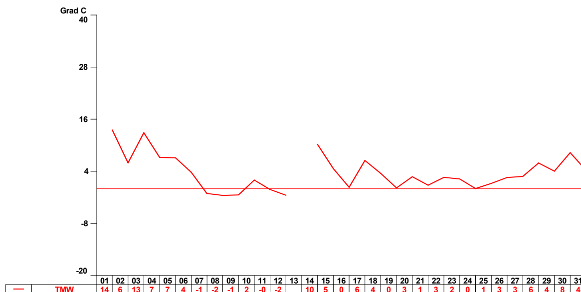
Abbildung 7: Eisenstadt Lufttemperatur
