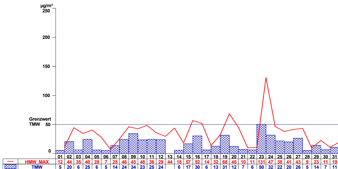
Abbildung 4: Eisenstadt PM 10
