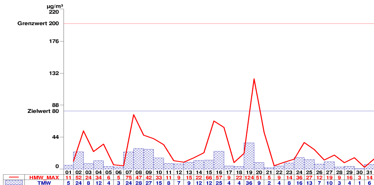
Abbildung 19: Kittsee NO 2
