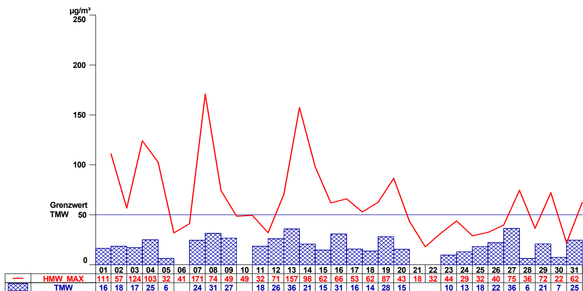
Abbildung 12: Oberschützen PM 10
