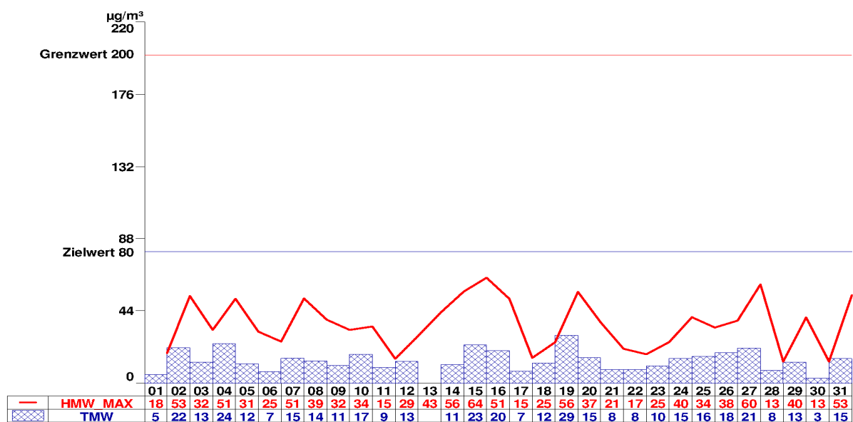
Abbildung 3: Eisenstadt NO 2
