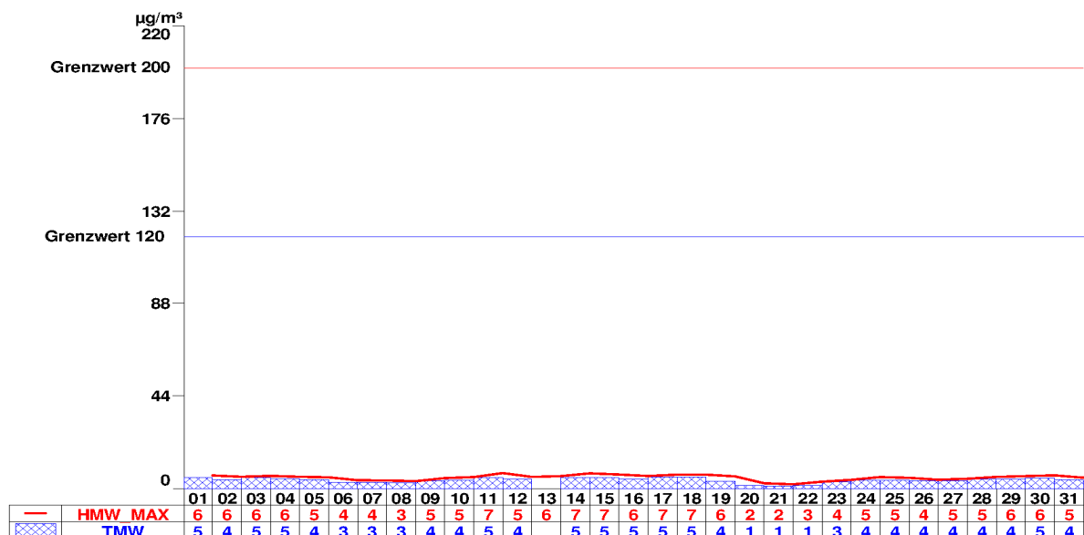
Abbildung 2: Eisenstadt SO 2
