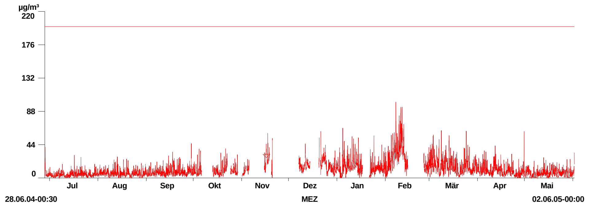
Abbildung 13: Stickstoffdioxid (Halbstundenmittelwerte)
