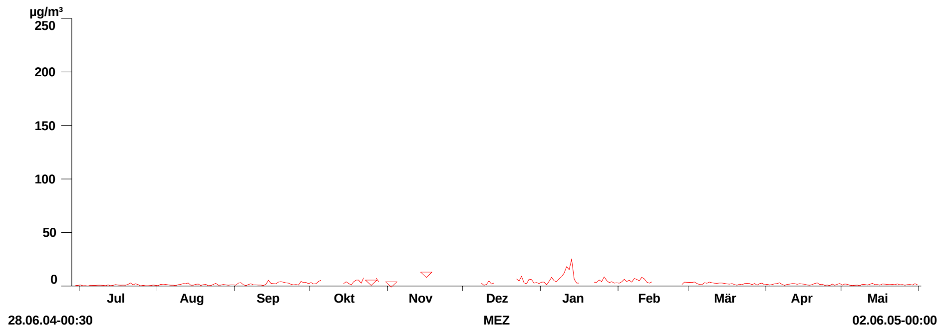
Abbildung 12: Stickstoffmonoxid (Tagesmittelwerte)
