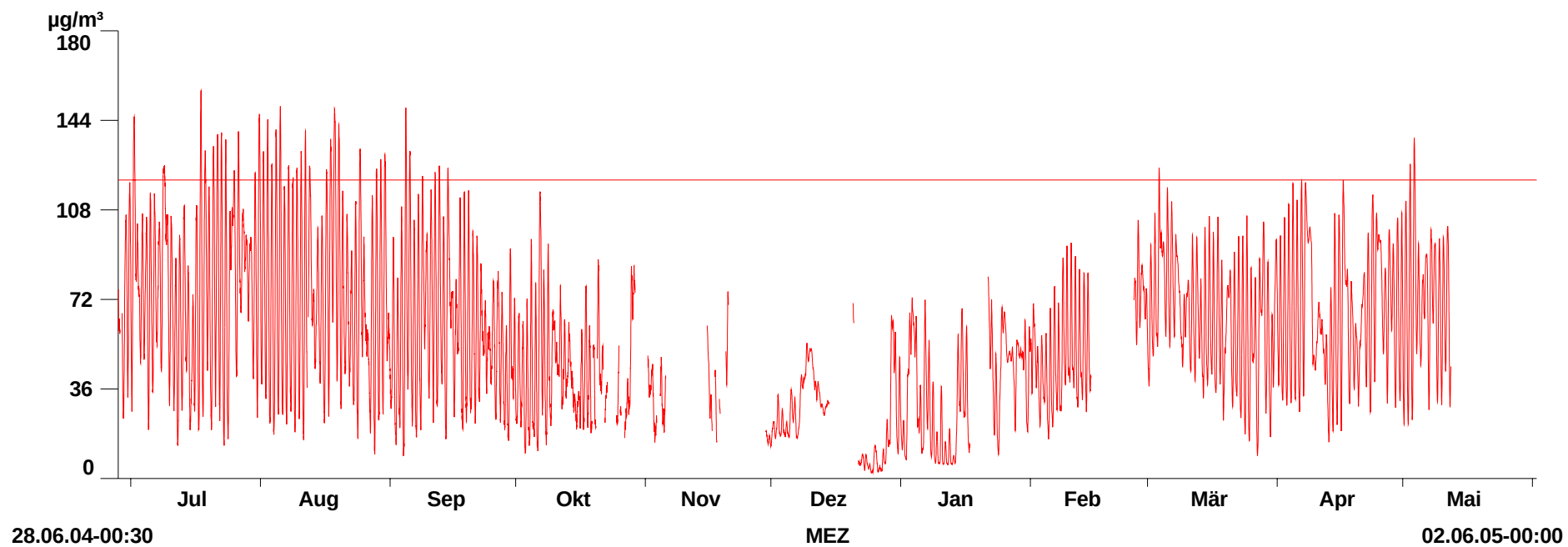
Abbildung 11: Ozon (Achtstundenmittelwerte)
