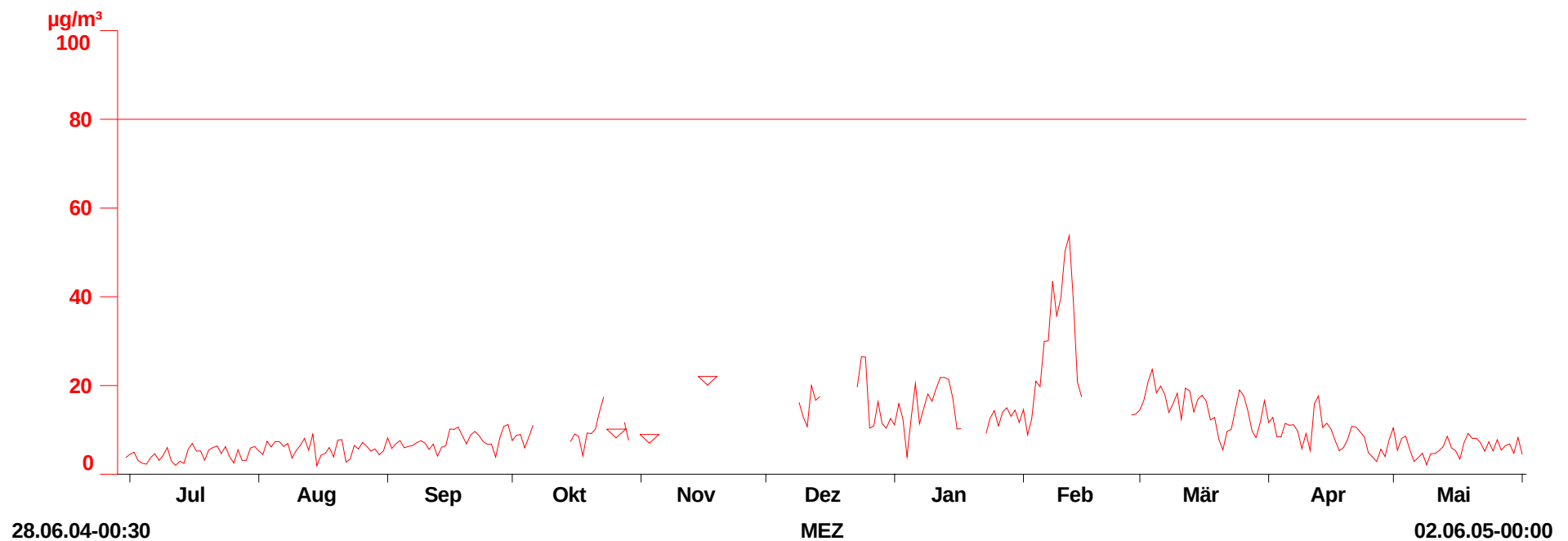
Abbildung 14: Stickstoffdioxid (Tagesmittelwerte)
