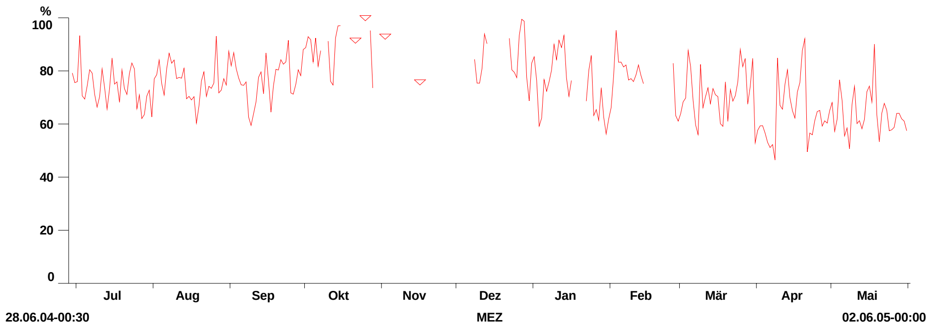
Abbildung 20: relative Luftfeuchte (Tagesmittelwerte)
