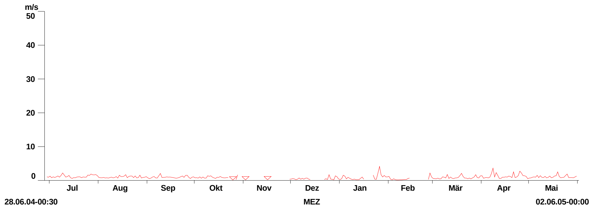
Abbildung 21: Windgeschwindigkeit (Tagesmittelwerte)
