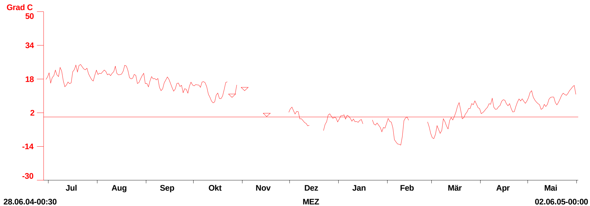
Abbildung 19: Temperatur (Tagesmittelwerte)
