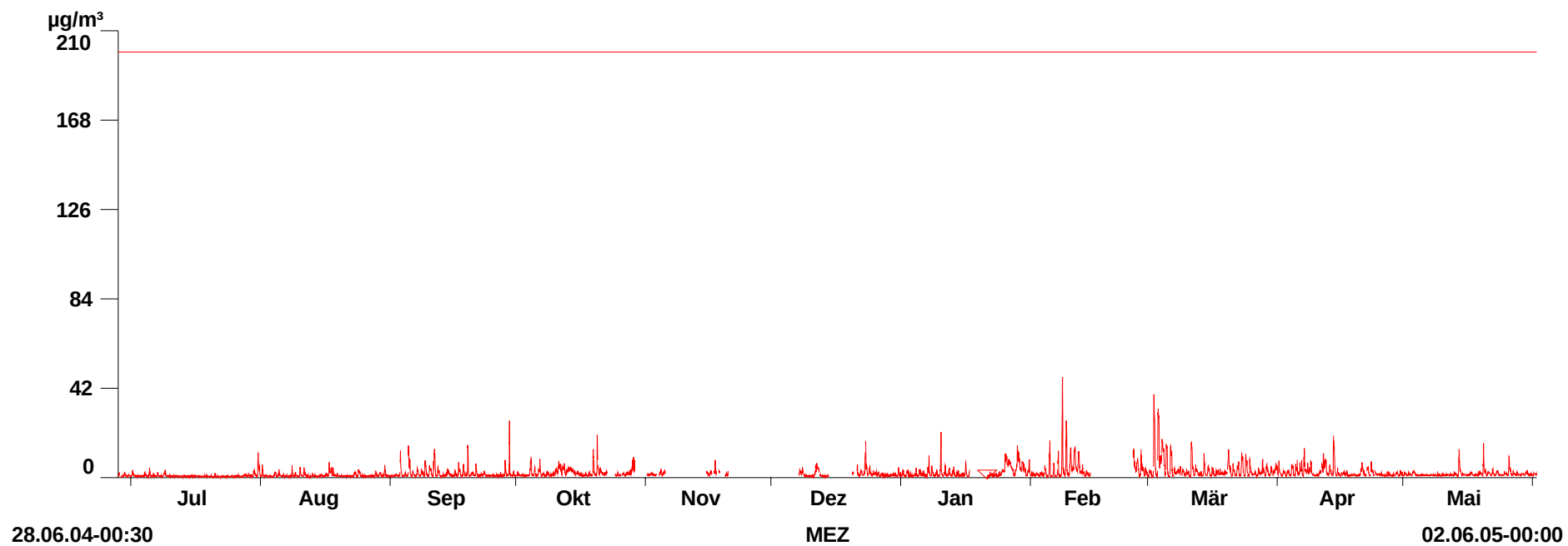
Abbildung 16: Schwefeldioxid (Halbstundenmittelwerte)
