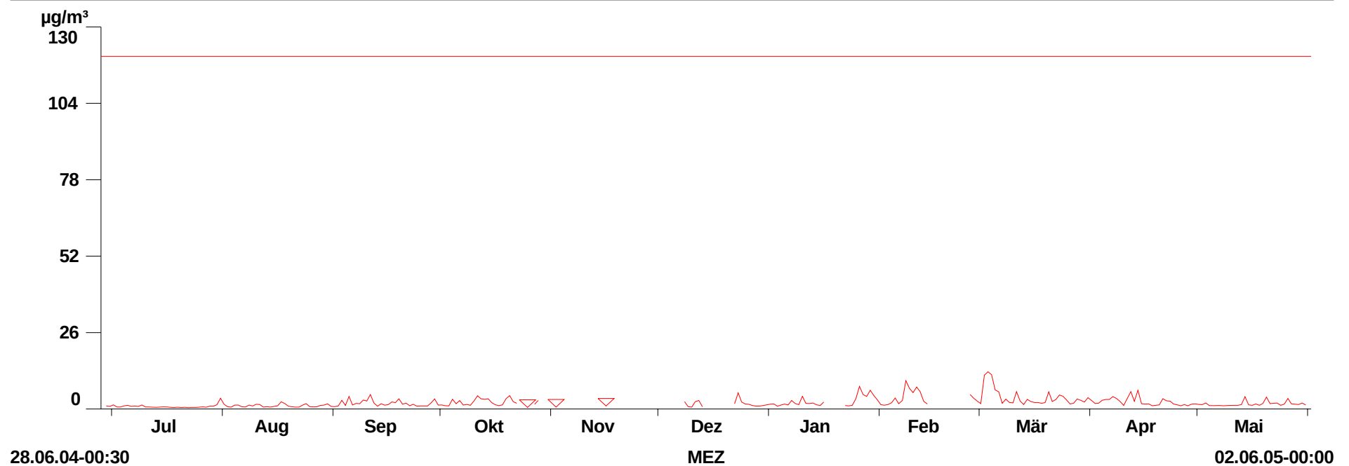
Abbildung 15: Schwefeldioxid (Tagesmittelwerte)
