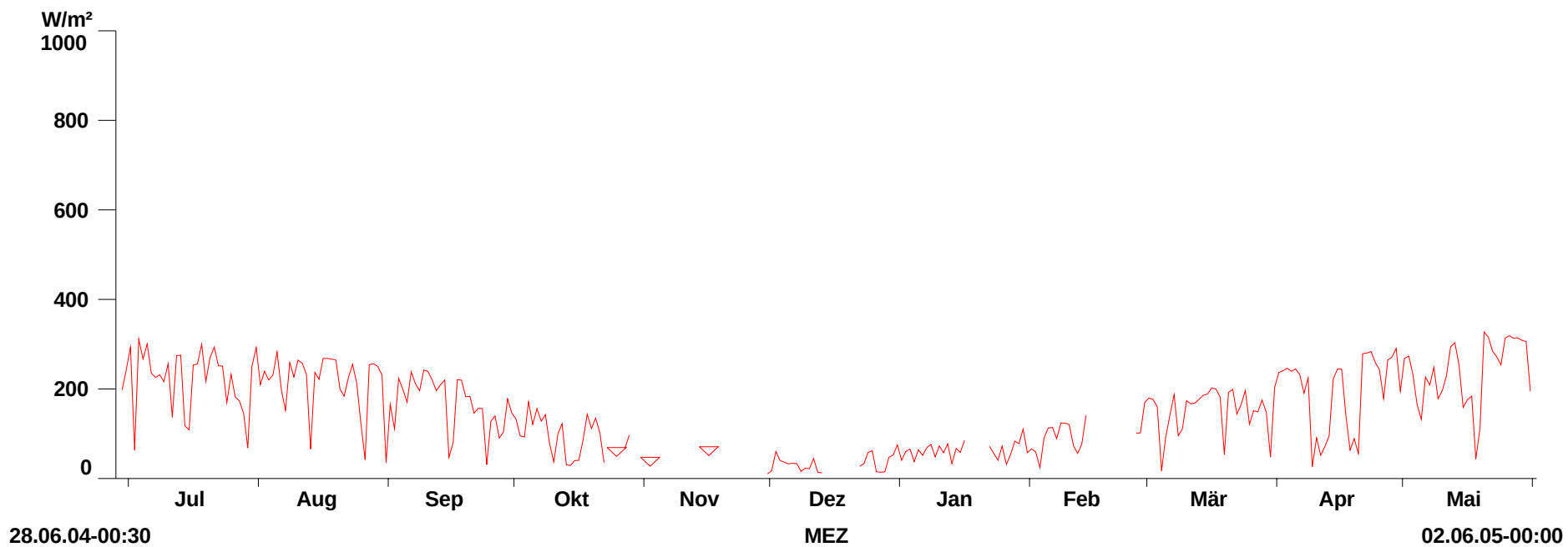
Abbildung 23: Globalstrahlung
