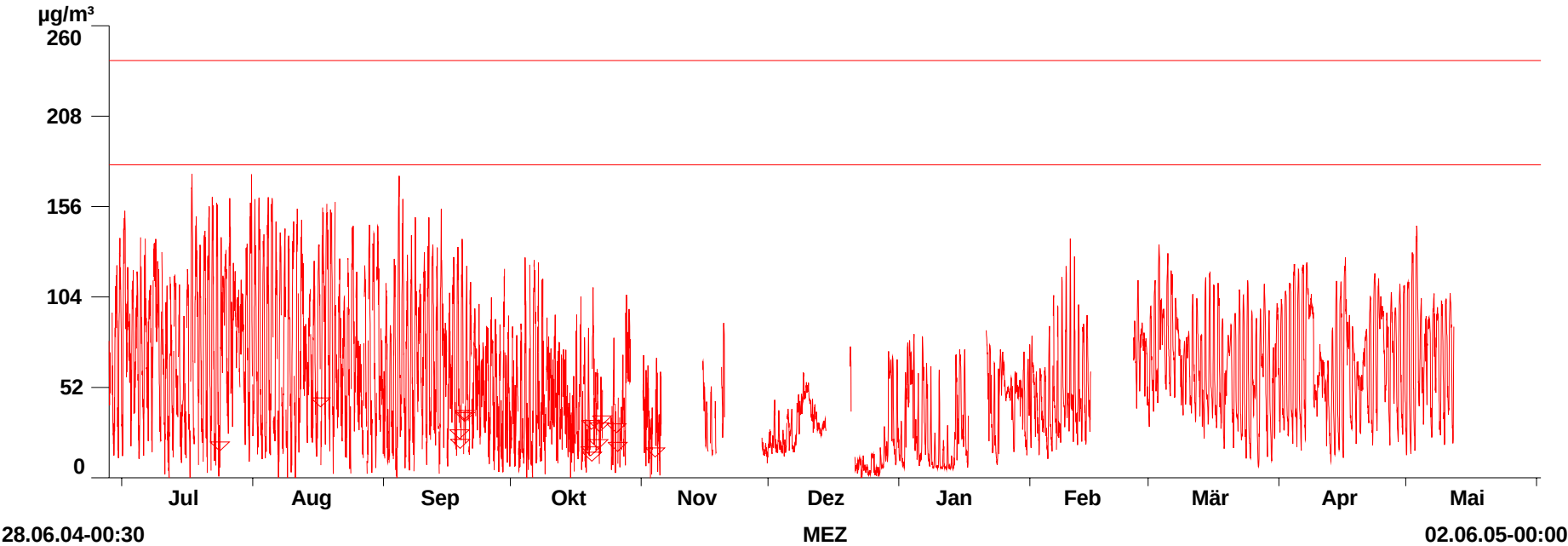
Abbildung 10: Ozon (Einstundenmittelwerte)
