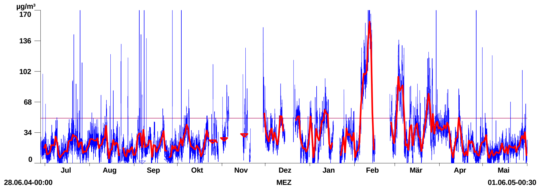
Abbildung 17: Feinstaub-PM10 (Tages- und Halbstundenmittelwerte)
