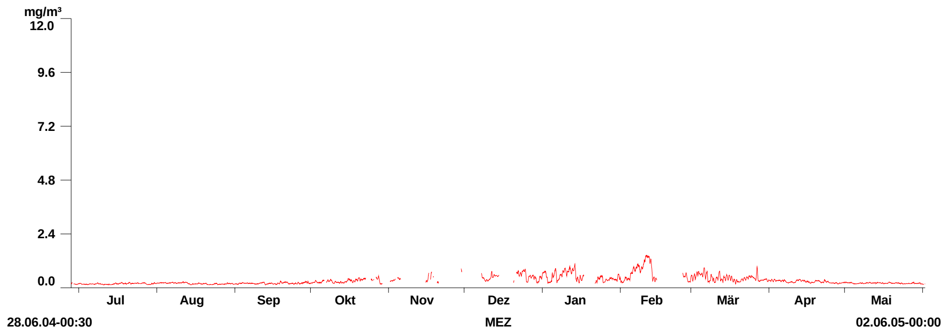
Abbildung 18: Kohlenmonoxid (Achtstundenmittelwerte)
